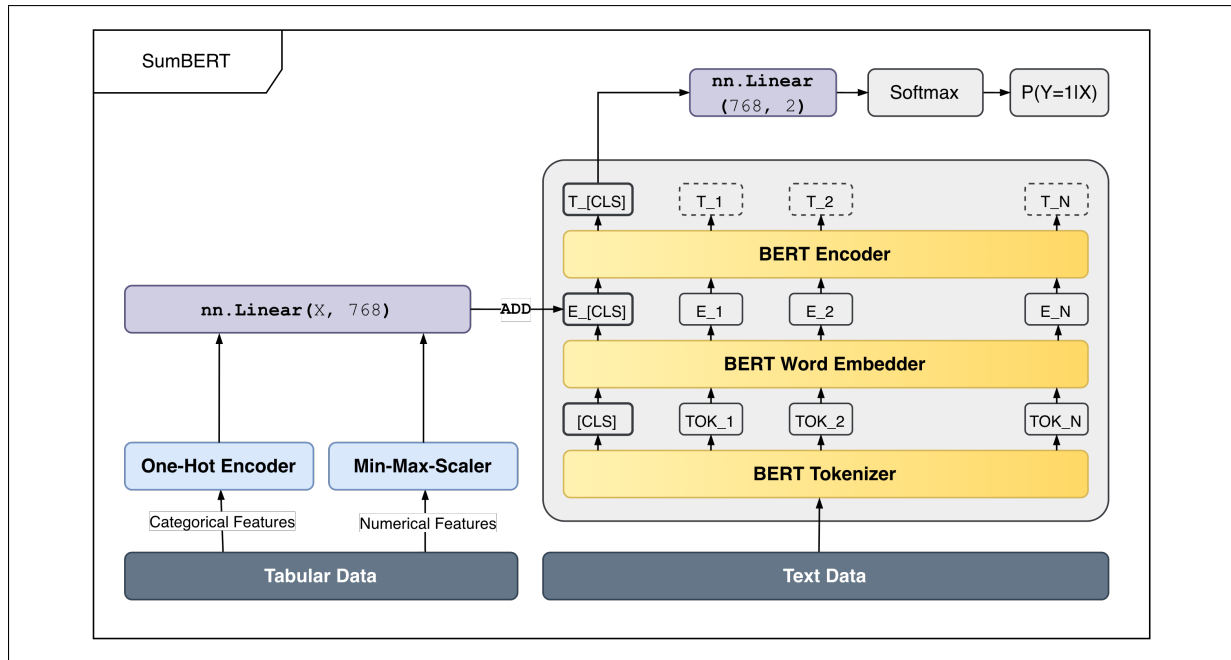
Abb. 1: Architektur von SumBERT: Addition der Tabellen-Repräsentation zum CLS-Token-Embedding vor dem Encoder. Quelle: [Fue24].
