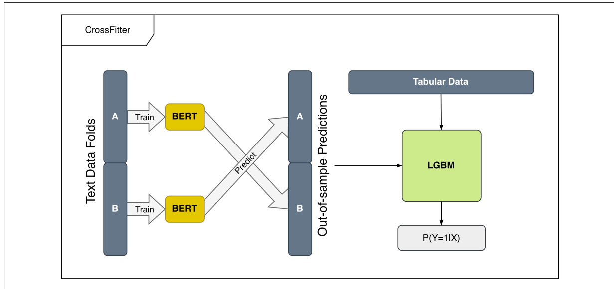
Abb. 8: Schematische Darstellung der CrossFitter-Modellarchitektur im produktiven Einsatz. Quelle: [Fue24].
