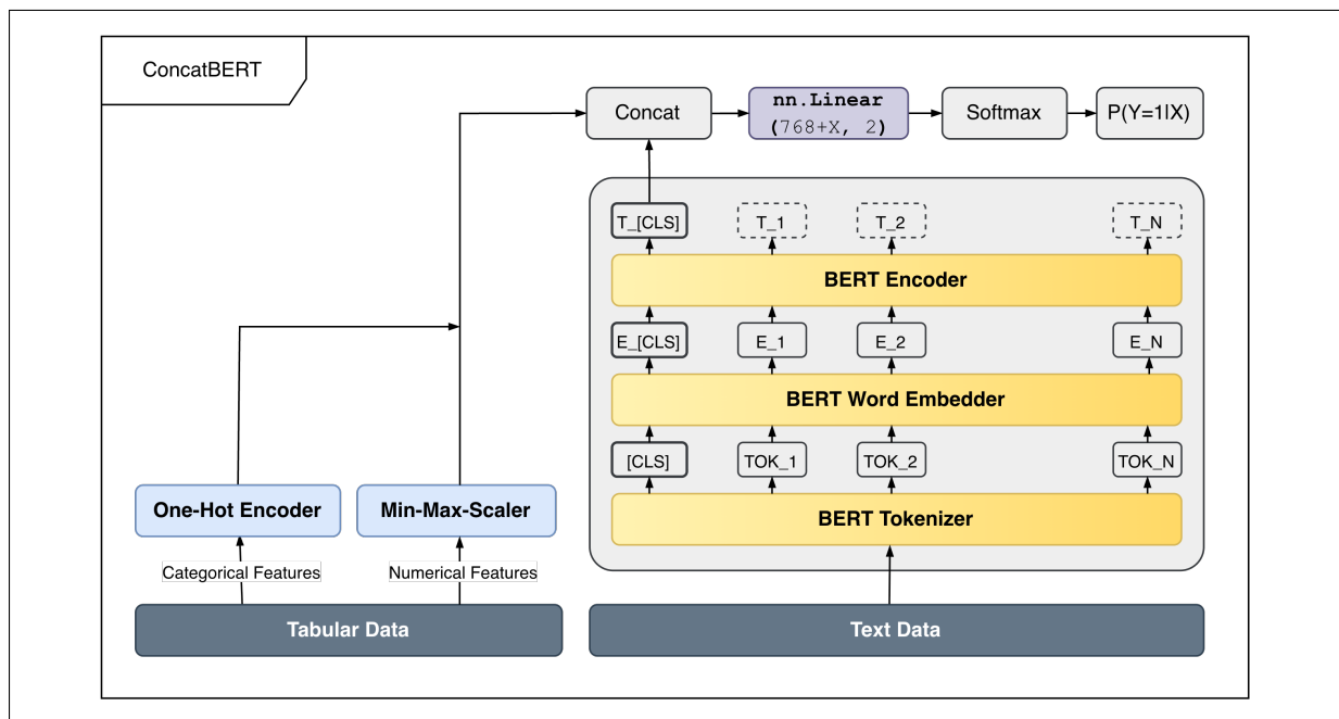
Abb. 2: Architektur von ConcatBERT: Konkatenation der Tabellen-Features mit dem Output des BERT-Encoders. Quelle: [Fue24].
