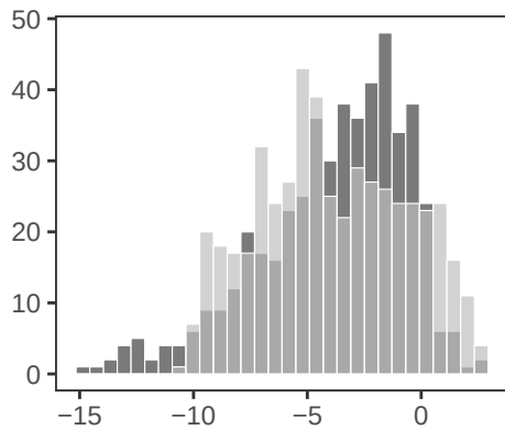
Binomial
