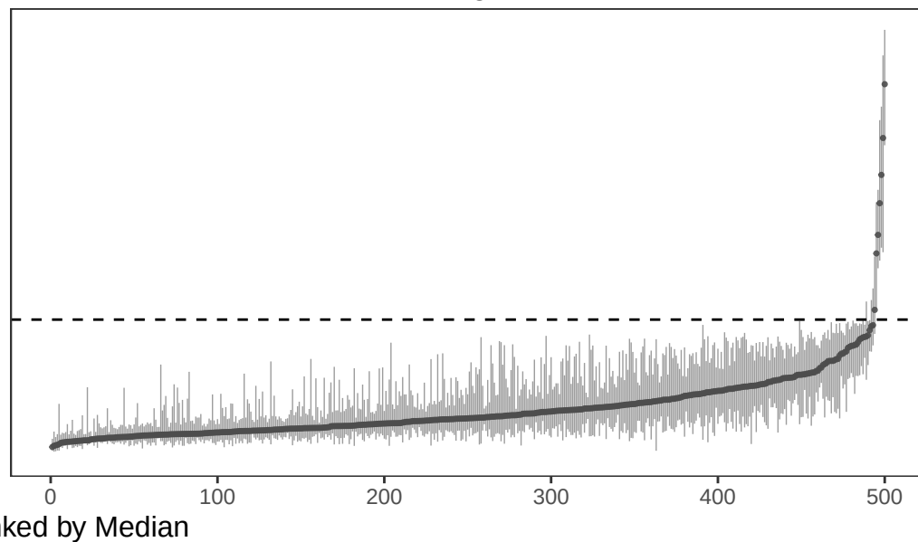
Integer
