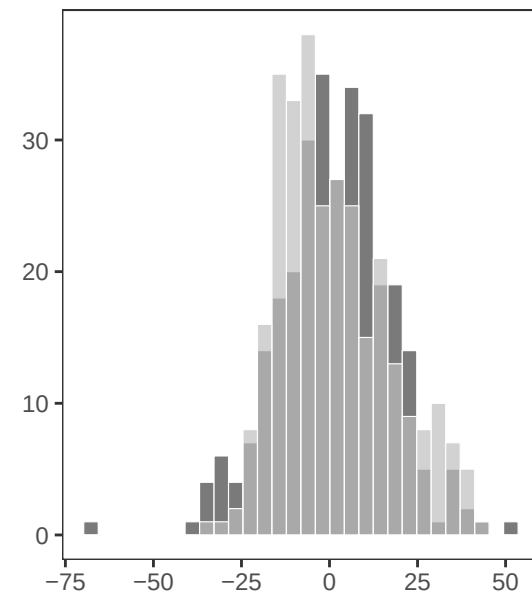
y Marginal
