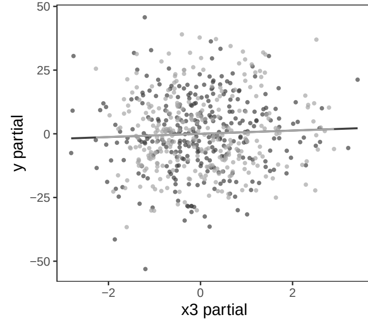
y Marginal
