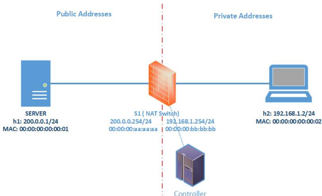
Figura 1: Topología Base
