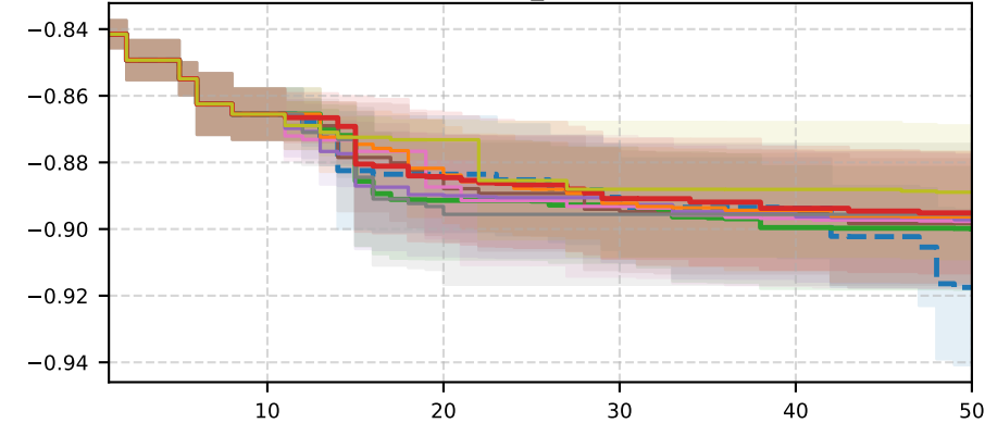
rbv2_1067
