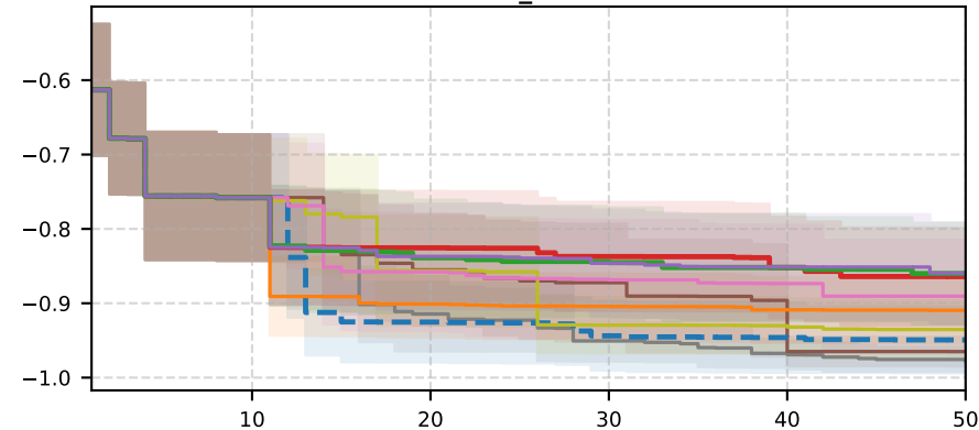
rbv2_1479
