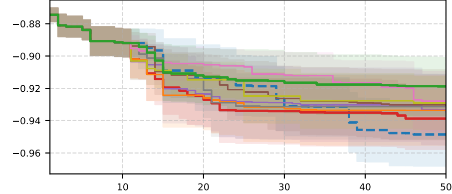
rbv2_1050
