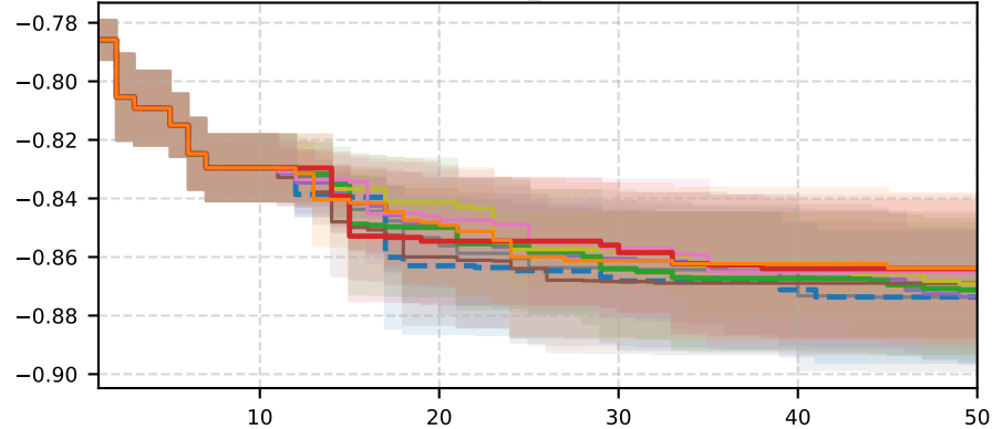
rbv2_1053
