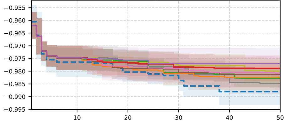
rbv2_1056
