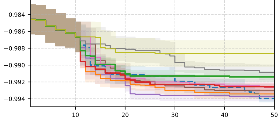
rbv2_1040
