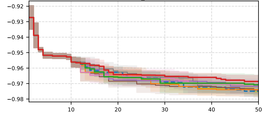
rbv2_1111
