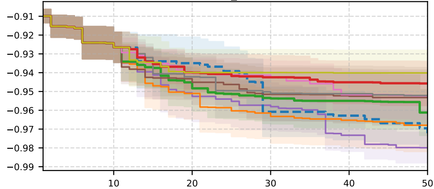
rbv2_1068
