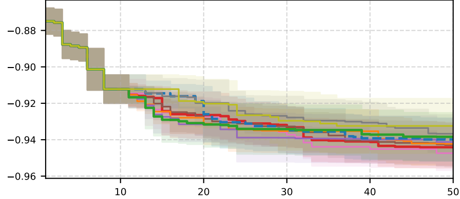
rbv2_1049
