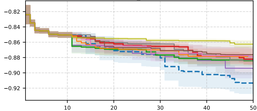
rbv2_1063
