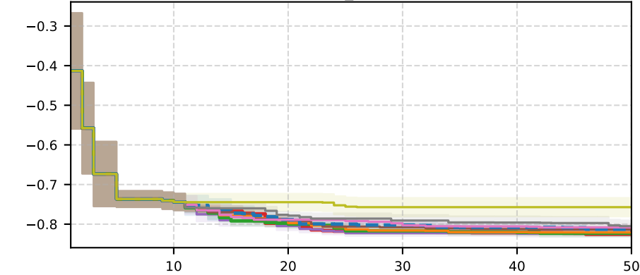
rbv2_1457
