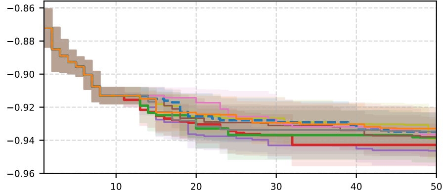
rbv2_1461
