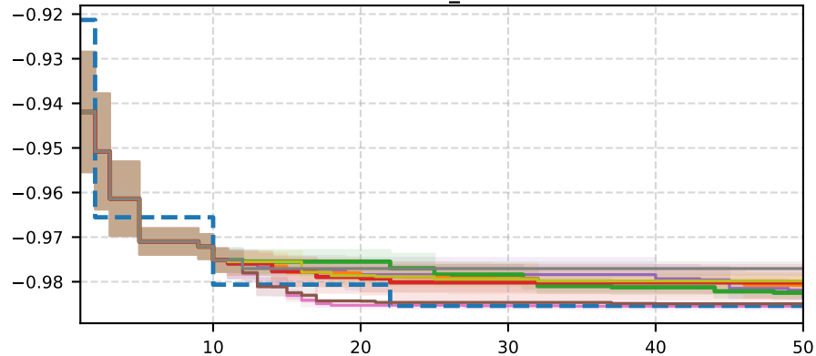
rbv2_15
