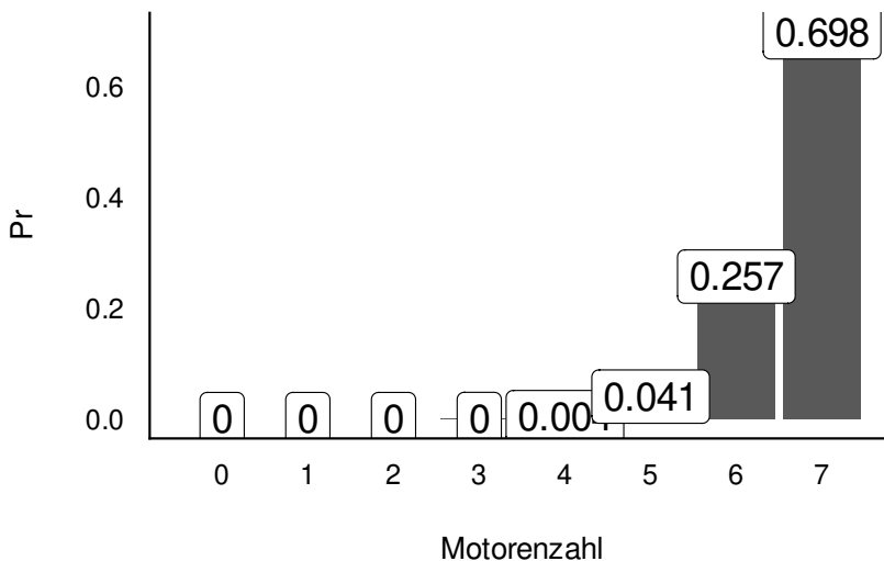
Abbildung 6.6: Wahrscheinlichkeit, dass genau k = 0..7 Motoren laufen
