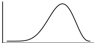
posterior
