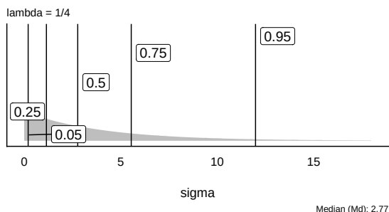
(d) lambda = 1/4
