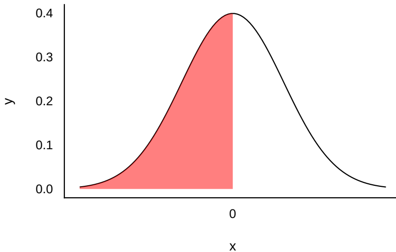
Abbildung 15.2: Verteilungsfunktion F(x=0)=1/2
