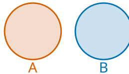
Abbildung 4.6: Zwei disjunkte Ereignisse, dargestellt durch überlappungsfreie Kreise
