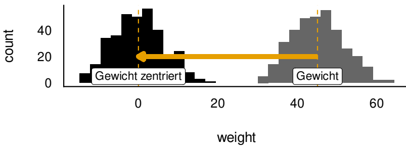
Abbildung 10.5: Das Zentrieren ändert die Verteilungsform nicht, sondern „schiebt“ die Verteilung nur zur Seite. Der resultierende Mittelwert ist dann Null. Die zentrierten Werte zeigen, wie weit ein Messwert vom Mittelwert entfernt ist (hier in der Einheit kg).
