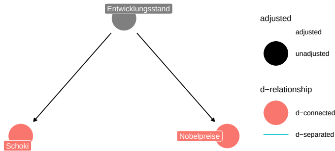
Abbildung 13.14: Macht Schokolade Nobelpreise?
