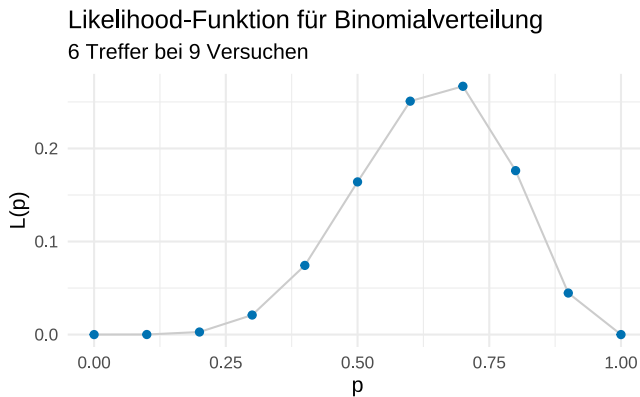
Abbildung 7.6: Die Likelihood-Funktion für x=6 Treffer, bei n=9 Würfeln, für eine binomialverteilte Zufallsvariable (mit 11 Parameterwerten: 0, 0.1, 0.2, ..., 1): Die Parameterwerte um 0.7 herum sind am plausibelsten.
