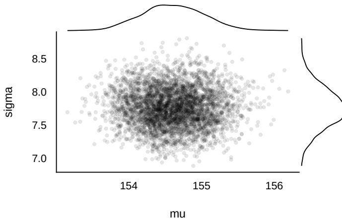
Abbildung 9.8: Die Postverteilung in unterschiedlicher Darstellung
