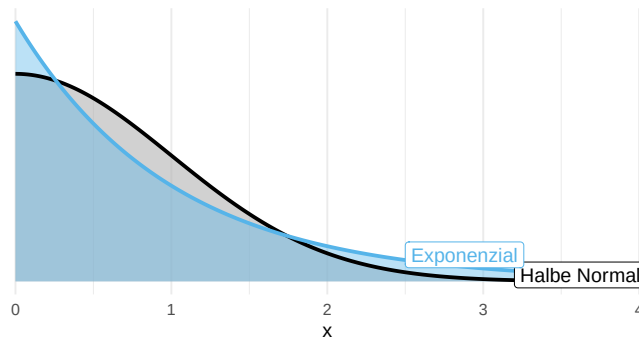
Abbildung 6.8: Exponentialverteilung (blau, Rate = 1) vs. halbe Normalverteilung (sd = 1)
