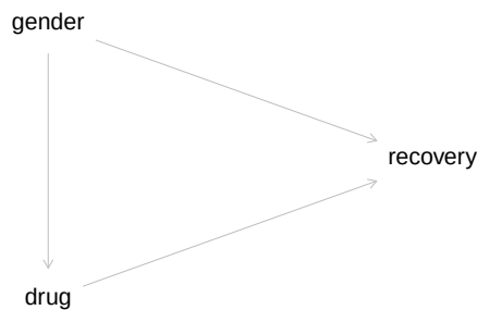
Abbildung 13.1: Zwei direkte Effekte (gender, drug) und ein indirekter Effekt (gender über drug) auf recovery
