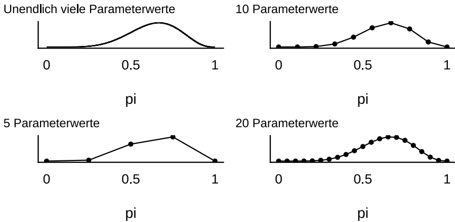
Abbildung 7.12: Die Post-Verteilung zunehmend mehr Parameterwerte in der Bayesbox. Je mehr Parameterwerte, desto ‚glatter‘ wird die Verteilung.
