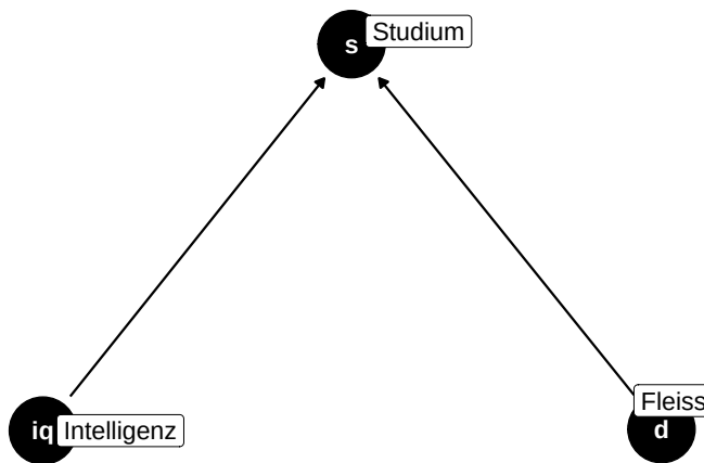
Abbildung 14.5: Kollisionsstruktur im Dag zur Studiumseignung
