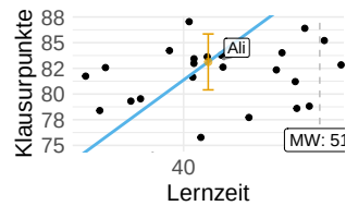
(b) Regressionsgerade mit Vorhersagebereich (und herangezoomt) für Ali
