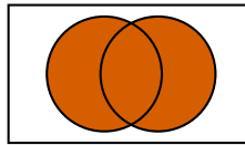
Abbildungung 4.11: A \cup B : Vereinigung zweier Mengen
