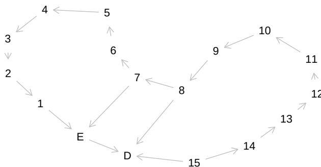
Abbildung 15.6: Ein DAG mit vielen Variablen
