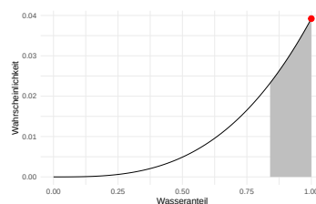
(b) Höchste-Dichte-Intervall (HDI)
