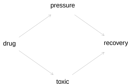
Abbildung 13.2: Drug hat keinen direkten, aber zwei indirekte Effekt auf recovery, einer davon ist heilsam, einer schädlich
