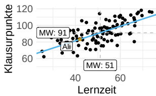
(a) Regressionsgerade mit Punkt-Vorhersage für Ali
