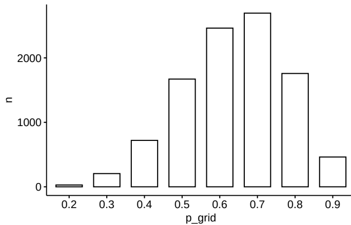
Abbildung 8.2: Stichprobenverteilung auf Basis von Stichproben
