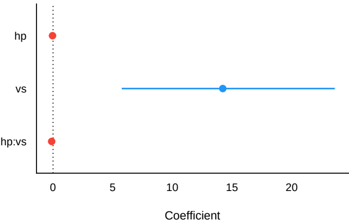
Abbildung 15.3: Parameter von m2 visualisiert
