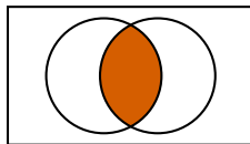
Abbildung 4.13: A \cap B : Schnitt zweier Mengen
