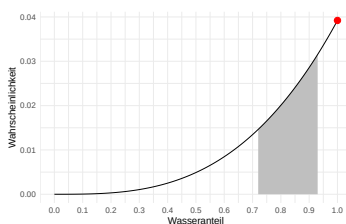
(a) Perzentilintervall (PI)
