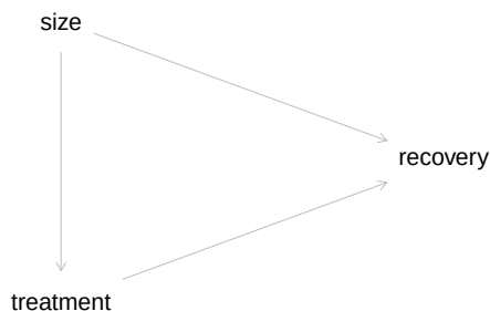
Abbildung 13.3: DAG zur Nierenstein-Studie
