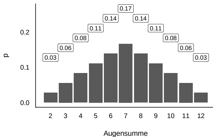
Abbildung 4.25: Wahrscheinlichkeitsverteilung der Zufallsvariable „Augenzahl im zweifachen Würfelwurf“
