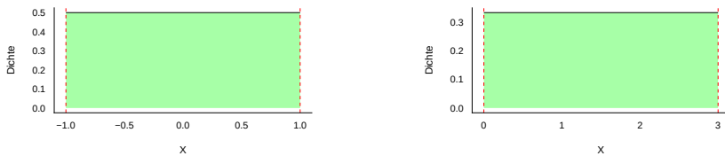
(a) Beispiel a: Gleichverteilung min=-1, max=1. Dichte: 1/2 (b) Beispiel b: Gleichverteilung min=0, max=3. Dichte: 1/3
