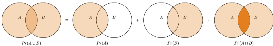
Abbildung 5.2: Der allgemeine Additionssatz gibt die Wahrscheinlichkeit, dass mindestens eines der beiden Ereignisse eintritt.
