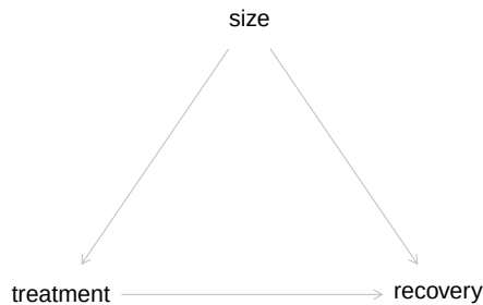
Abbildung 13.4: DAG zur Nierenstein-Studie in zweiter Darstellungsform
