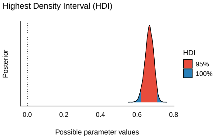
Abbildung 11.6: Die Verteilung von R-Quadrat im Modell m_penguins_species
