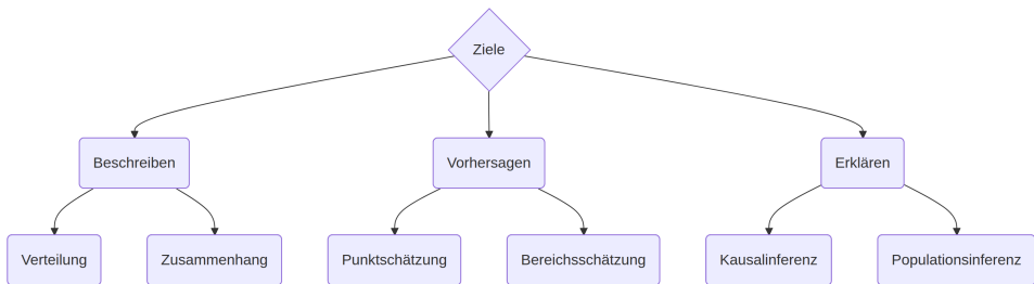
Abbildung 2.1: Eine Einteilung zentraler Ziele von statistischen Analysen
