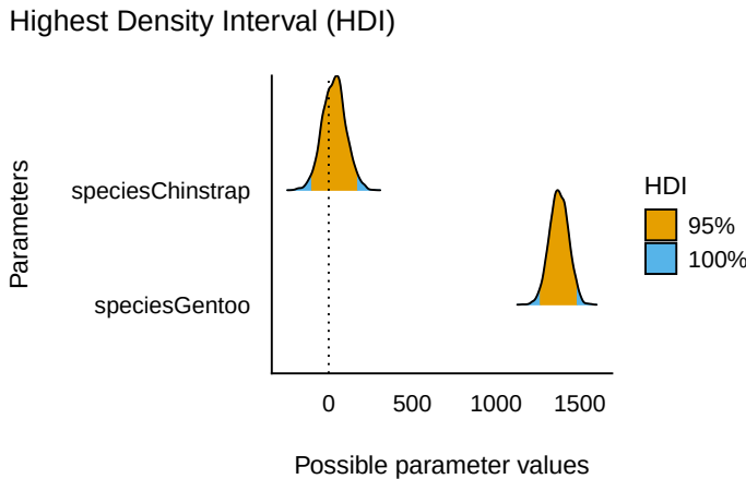
Abbildung 12.14: Effekt der UV: Unterschiede zur Referenzgruppe (95%-HDI)
