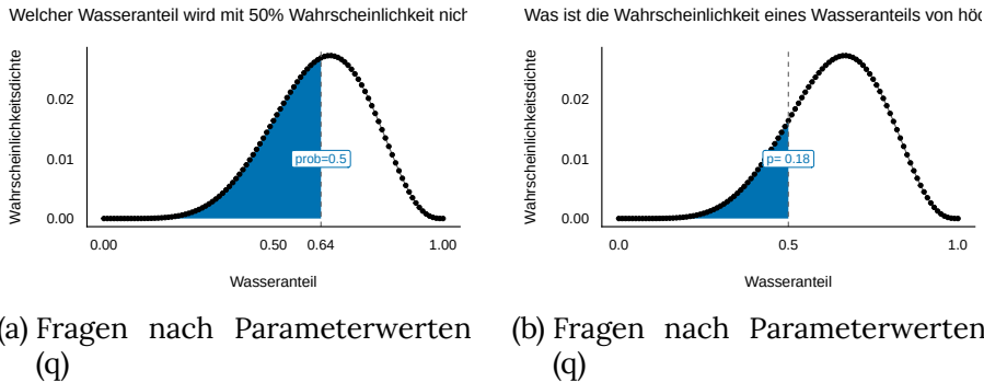
Abbildung 8.5: Unterschied zwischen Fragen nach Wahrscheinlichkeiten (p) und Fragen nach Parameterwerten (q)
