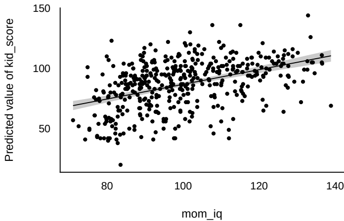
Abbildung 12.6: Die geschätzten Erwartungswerte von m10.2 visualisiert
