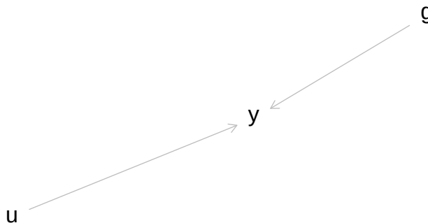
Abbildung 12.11: DAG für y \sim g
