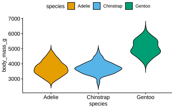
Abbildung 12.13: Verteilung des Körpergewichts dreier Arten von Pinguinen – Geom Violine
