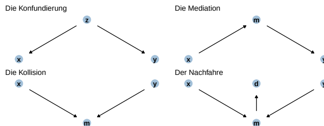
Abbildung 14.12: Die vier Atome der Kausalinferenz
