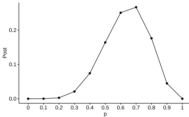
Abbildung 7.11: Die Post-Verteilung visualisiert. Die Post-Wahrscheinlichkeit ist am höchsten bei p=0.7
