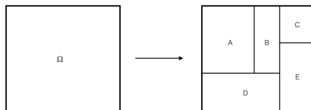
Abbildung 4.3: Zerlegung des Grundraums in ein vollständiges Ereignissystem
