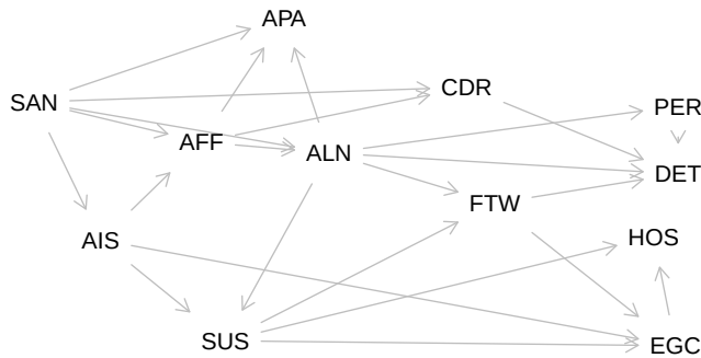
Abbildung 15.7: Ein DAG zu den Symptomen der Schizophrenie
