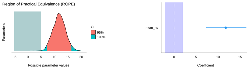
(a) Diagramm mit rope(m10.1) |> plot() (b) Diagramm mit parameters(m10.1) |> plot()
