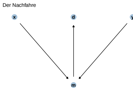
Abbildung 14.15: Ein Nachfahre verhält sich ähnlich wie sein Vorfahre...
