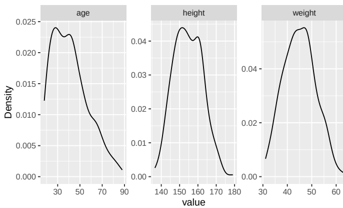
Abbildung 9.2: Verteilungen der Variablen im Kung-Datensatz. Größe und Gewicht sind recht symmetrisch bzw. normalverteilt; Alter ist rechtsschief.
