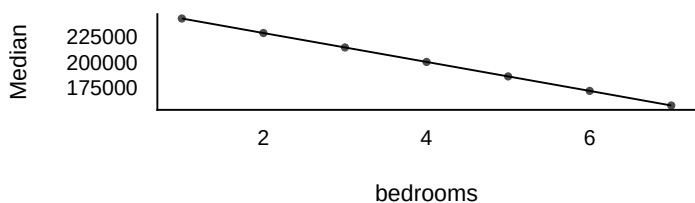
Abbildung 13.6: Hauspreis als Funktion der Zimmerzahl, laut m2
