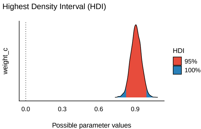
Abbildung 10.12: Die Parameter Gewicht (zentriert) Modells m_kung_starkes_beta1
