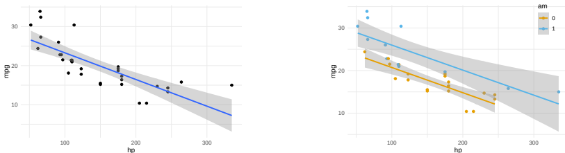
(a) Einfache Regression (eine UV: hp) (b) Multiple Regression (zwei UV: hp und am)
