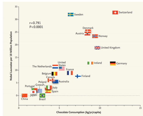
Abbildung 13.15: Je mehr Schoki, desto mehr Nobelpreise
