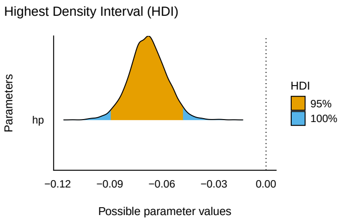
Abbildung 15.4: Post-Verteilung (HDI) von m3
