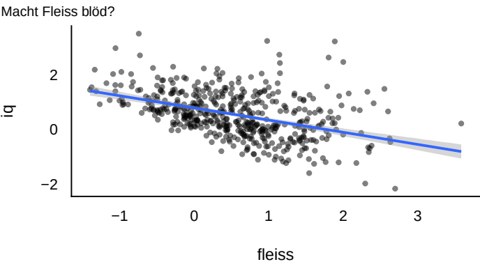
Abbildung 14.6: Der Zusammenhang von Fleiss und IQ
