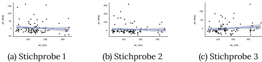
Abbildung 3.4: Regressionsanalysen mit verschiedenen Koeffizienten aufgrund der Zufälligkeit des Stichprobenziehens
