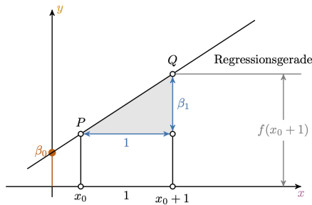
(a) Die eine Regression
