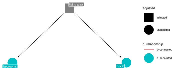
Abbildung 13.9: Durch Kontrolle von living area wird die Assoziation von price und bedrooms aufgehoben.
