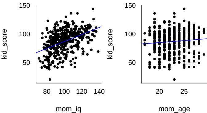
Abbildung 12.16: Zwei univariate Regressionen
