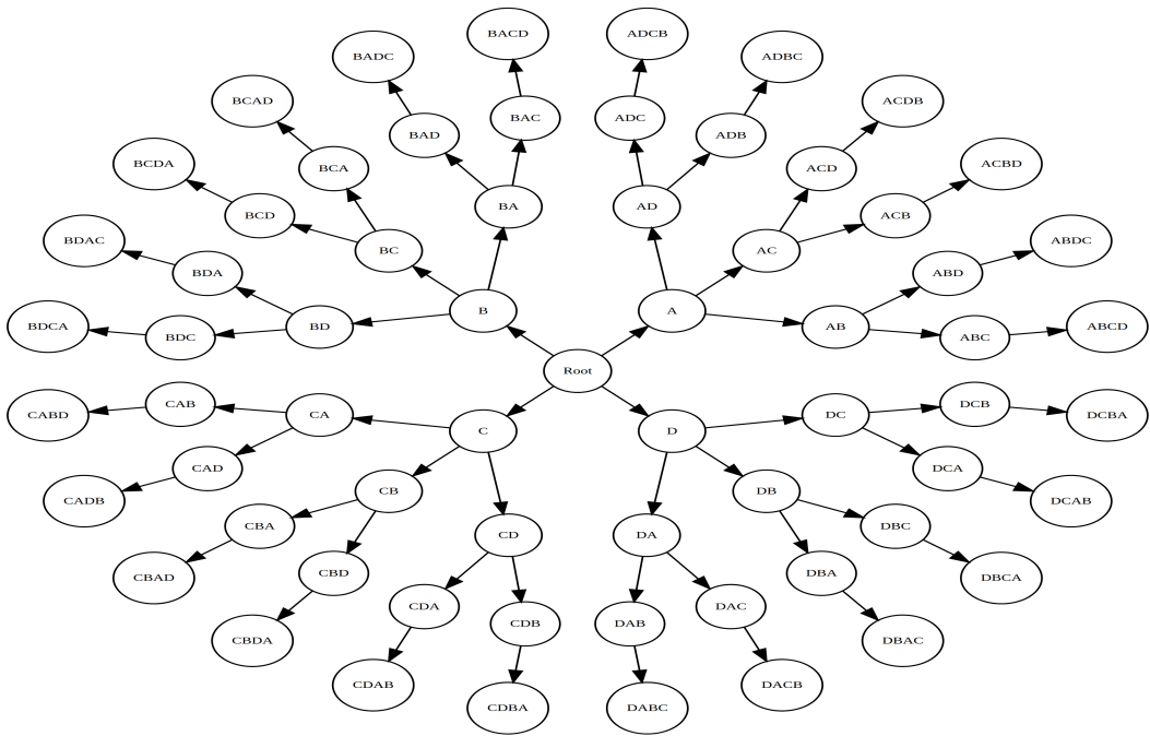
Abbildung 6.4: Sie wählen nacheinander 4 Freunde (A,B,C,D) aus. Wie viele Möglichkeiten gibt es dafür? Zuerst haben Sie 4 Möglichkeiten. Nachdem Sie den 1. Freund gewählt haben, haben Sie noch 3 weitere zur Auswahl. Dann noch 2 und schließlich bleibt der Letzte.
