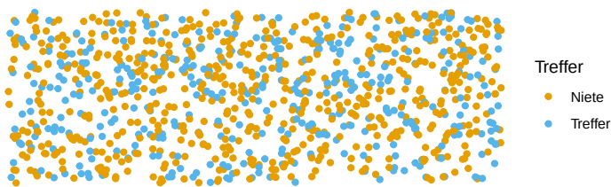
Abbildung 6.2: Ein Kästchen mit Losen, davon 2/5 Treffer und 3/5 Nieten
