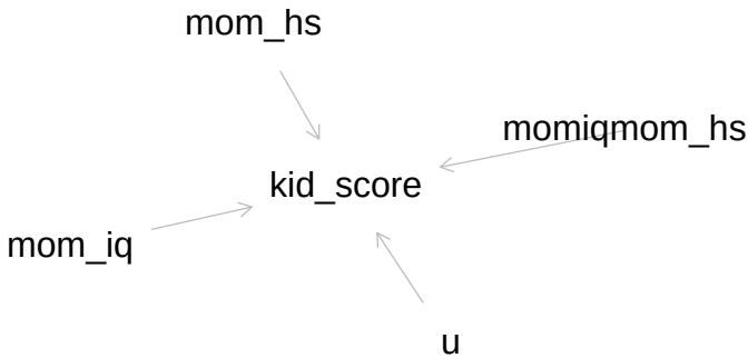
Abbildung 12.8: DAG für y \sim x + b + x:b
