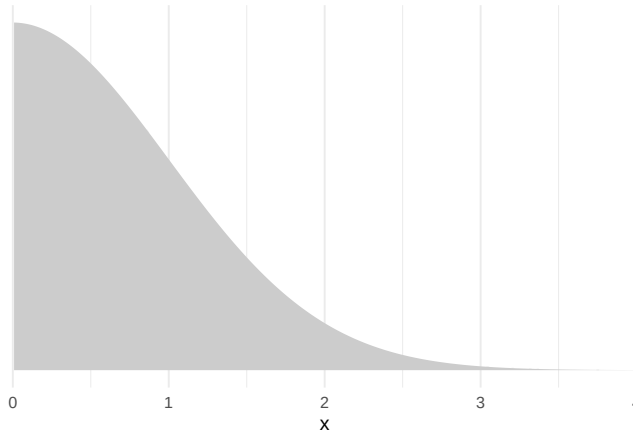
Abbildung 6.7: Die halbe Normalverteilung
