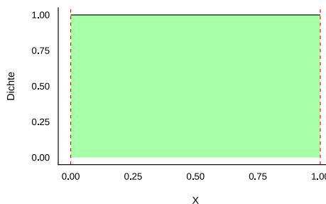
Abbildung 7.8: Gleichverteilung mit Parametern min=0 und max=1
