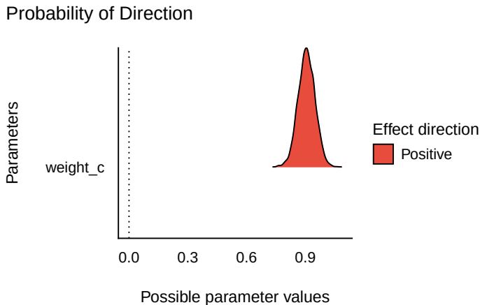
Abbildung 10.8: Diagramm zur Probability of Direction, Modell m_kung_starkes_beta1
