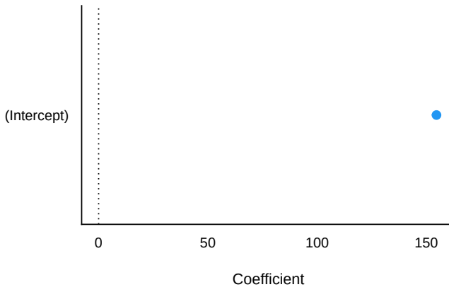
Abbildung 9.11: Parameter von m_kung , nur einer: der Intercept
