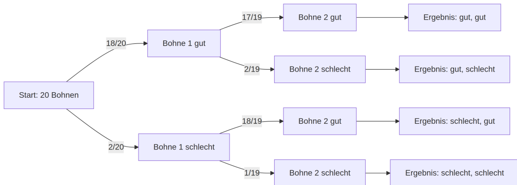
Abbildung 5.9: Baumdiagramm für ein ein zweistufiges Zufallsereignis: Bertie Botts Bohnen.
