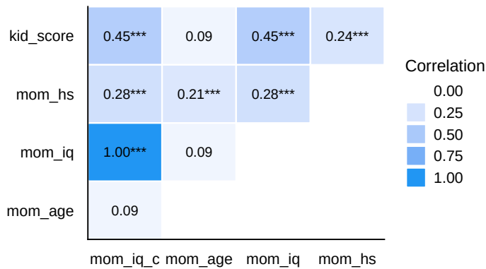
Abbildung 12.15: Visualisierung der Korrelationsmatrix als Heatmap
