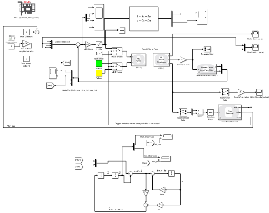
Figura 5: Integración del controlador LQR y el observador de estados.
