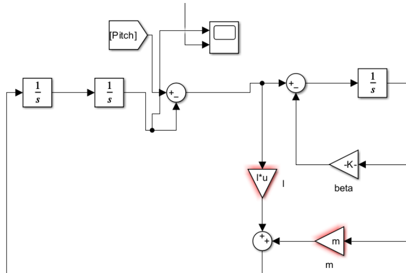
Figura 4: Arquitectura en Simulink del sistema LQR.
