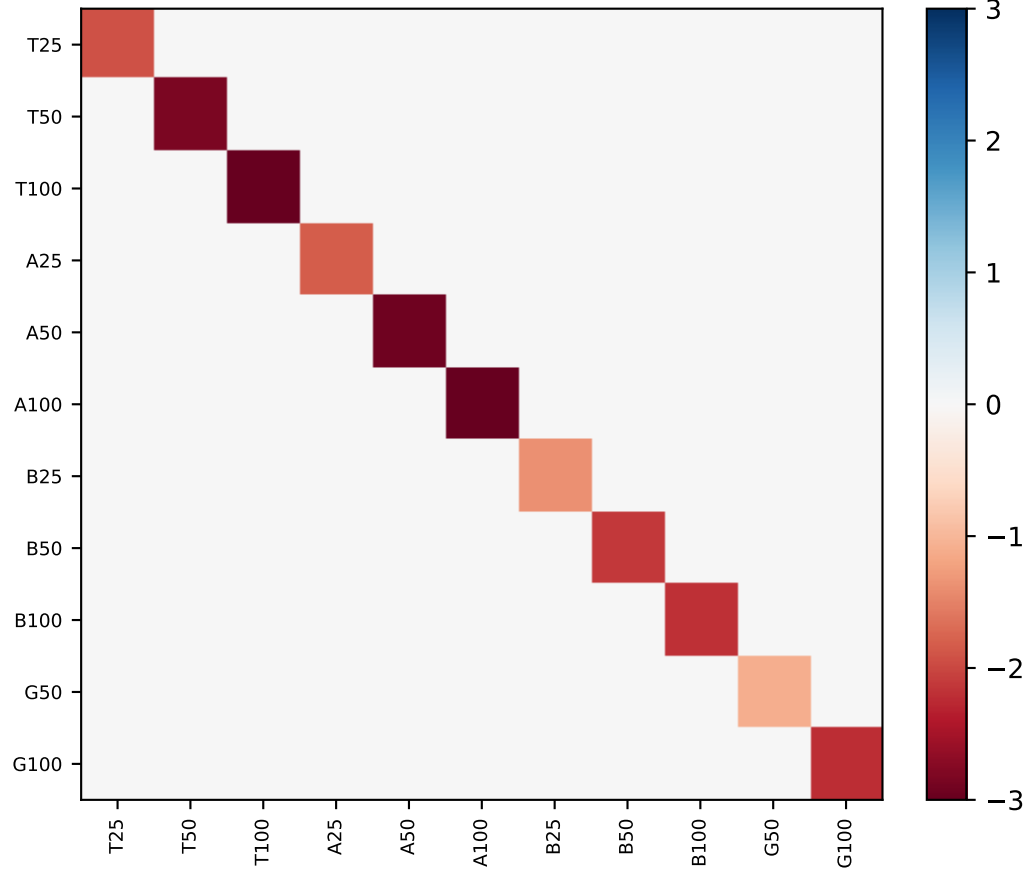
Elasticidades Logit (IV) -- 109/39
