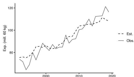
Figura 21: Ajuste del modelo. Exportaciones
