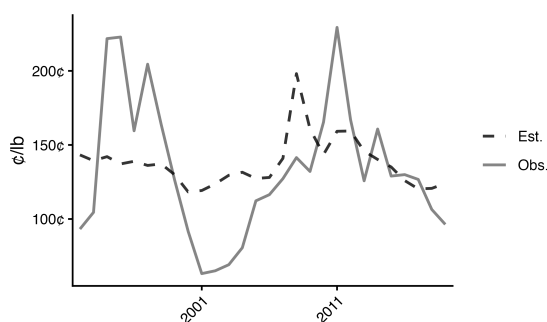
Figura 20: Ajuste del modelo. Precio del café
