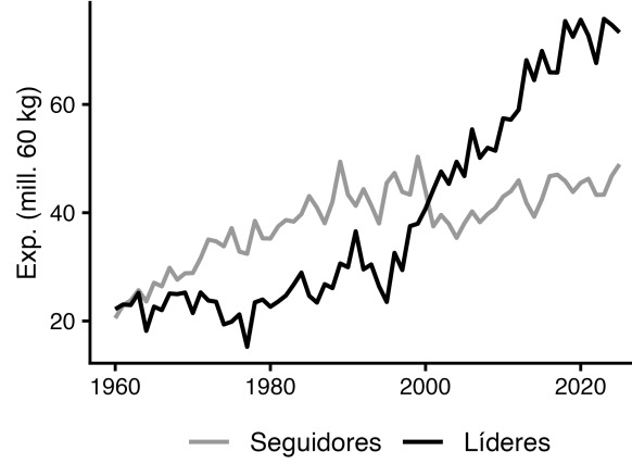
Figura 3: Exportaciones mundiales de café, por grupos de países
