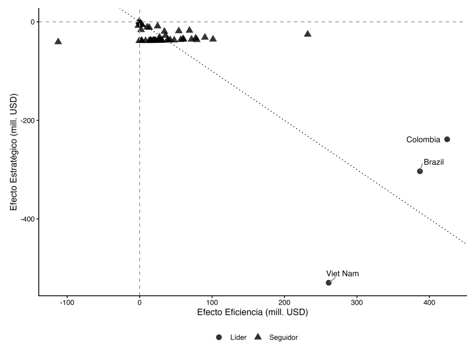
Figura 27: Descomposición del excedente total acumulado en 1990-2019, por país
