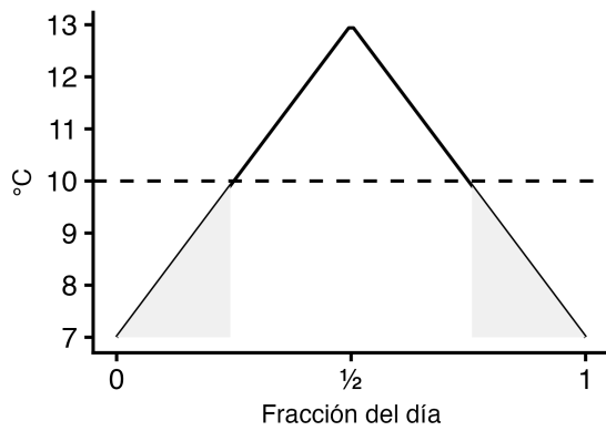
Figura 16: Escenario con exposición parcial al frío extremo
