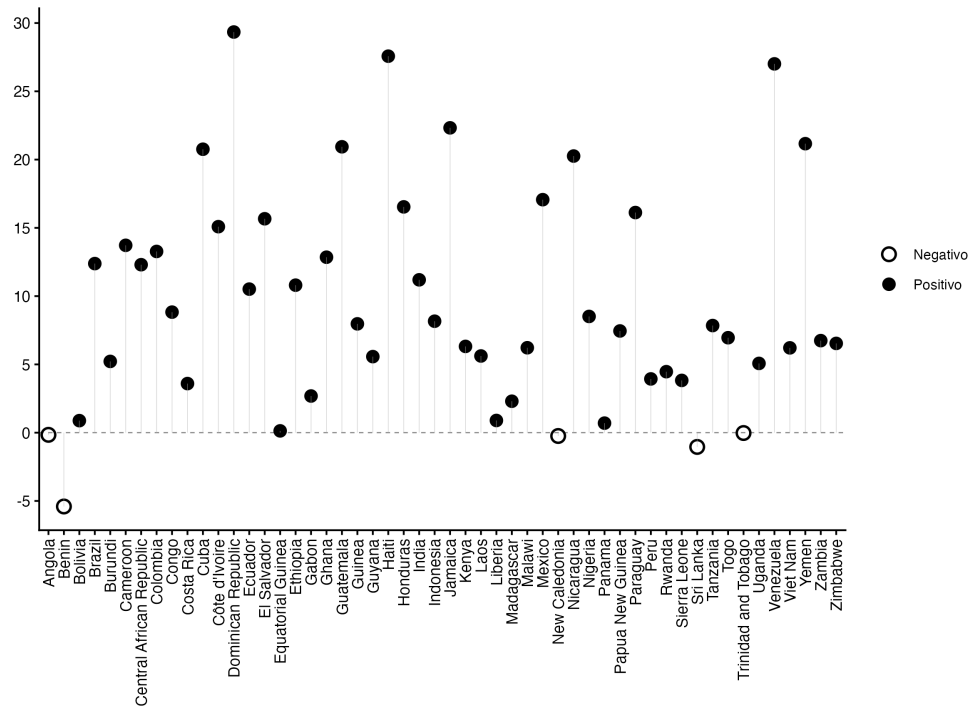
Figura 22: Promedio anual de días adicionales de estrés térmico (1970-1989 vs. 1990-2019)
