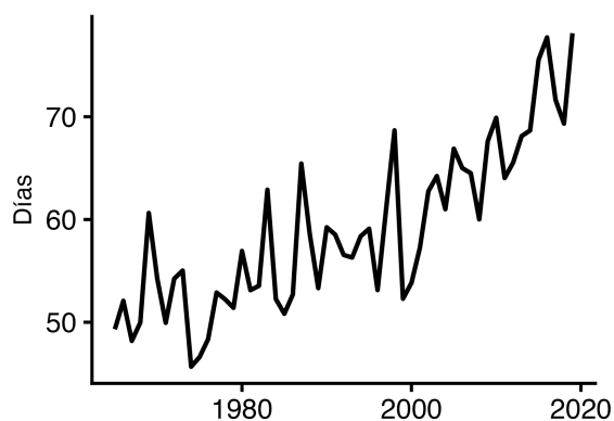
Figura 2: Exposición a temperaturas en extremo altas
