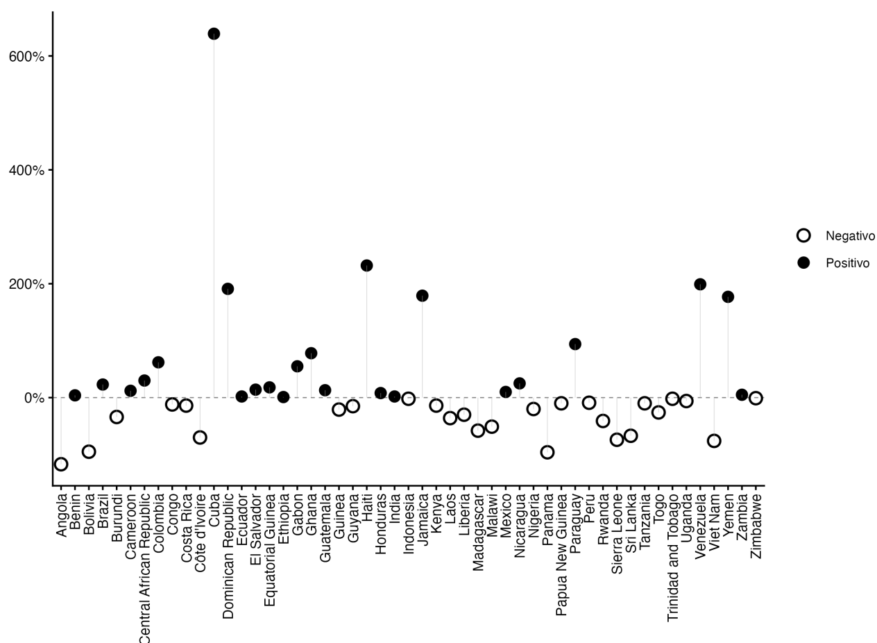
Figura 26: Cambio en el beneficio por país
