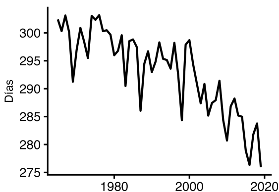
Figura 1: Exposición anual al rango óptimo de temperatura
