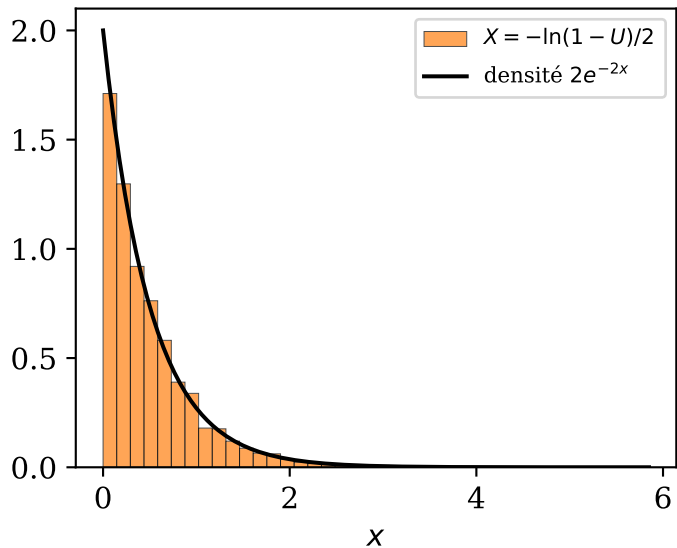
Transformation inverse : loi exponentielle
