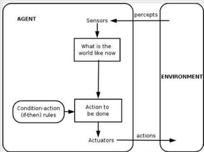
단순 반사 에이전트 다이어그램
