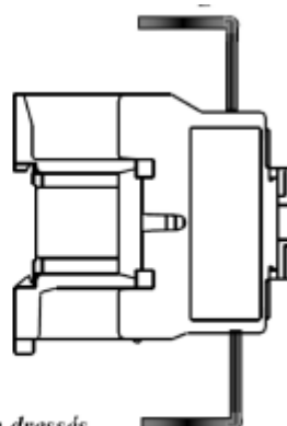
Fils bien dressés et non croisés
