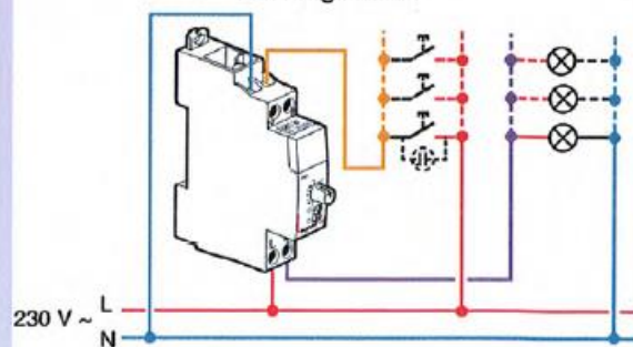
Montage 4 fils
