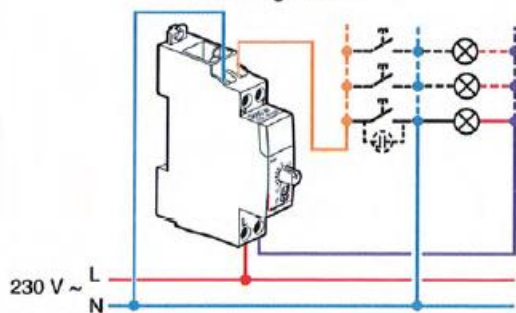
Montage 3 fils
