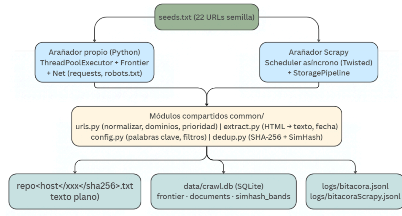
Figura 1. Arquitectura: dos motores de arañado sobre módulos de política y almacenamiento compartidos.
