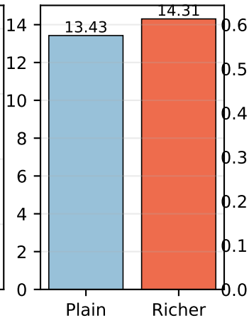
Sparseness
