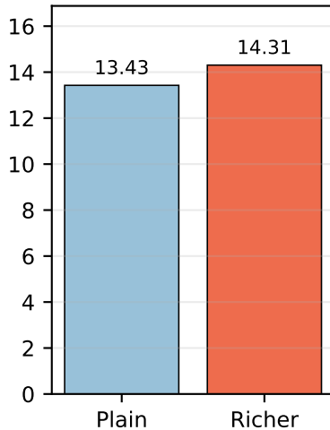
Sparseness
