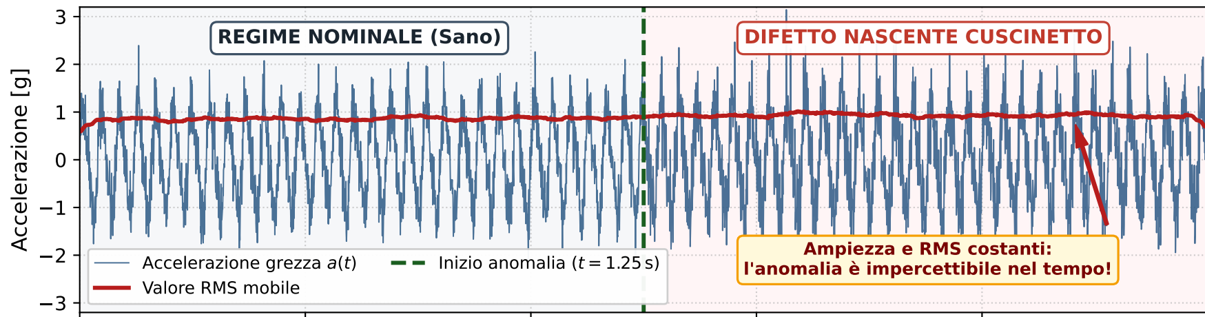
(a) Segnale vibrazionale nel dominio del tempo e indicatore RMS
