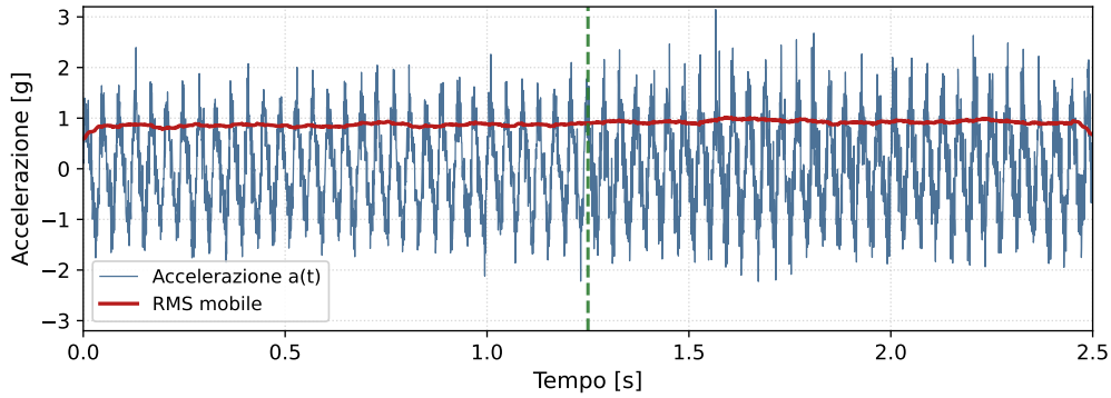
(a) Segnale con anomalia nel dominio del tempo
