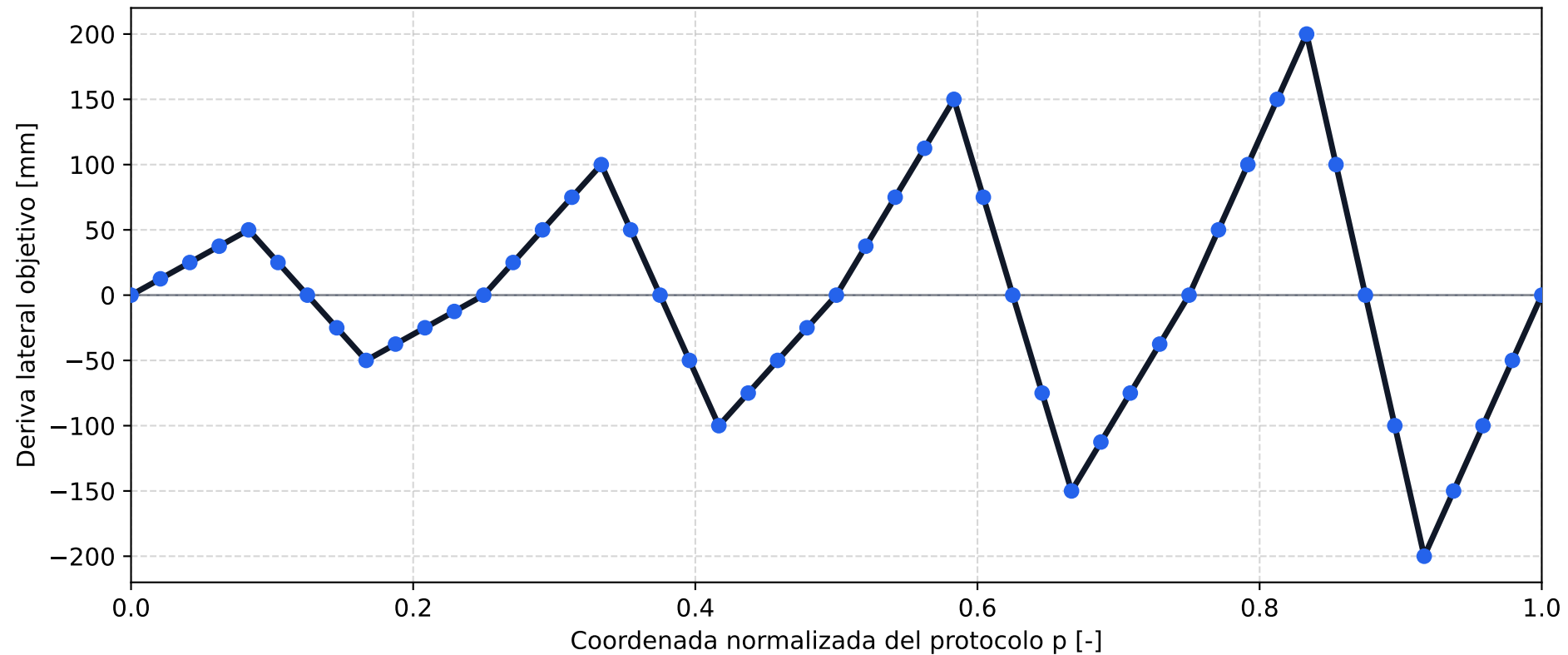
Protocolo cíclico de auditoría de la columna hasta \pm 200 mm
