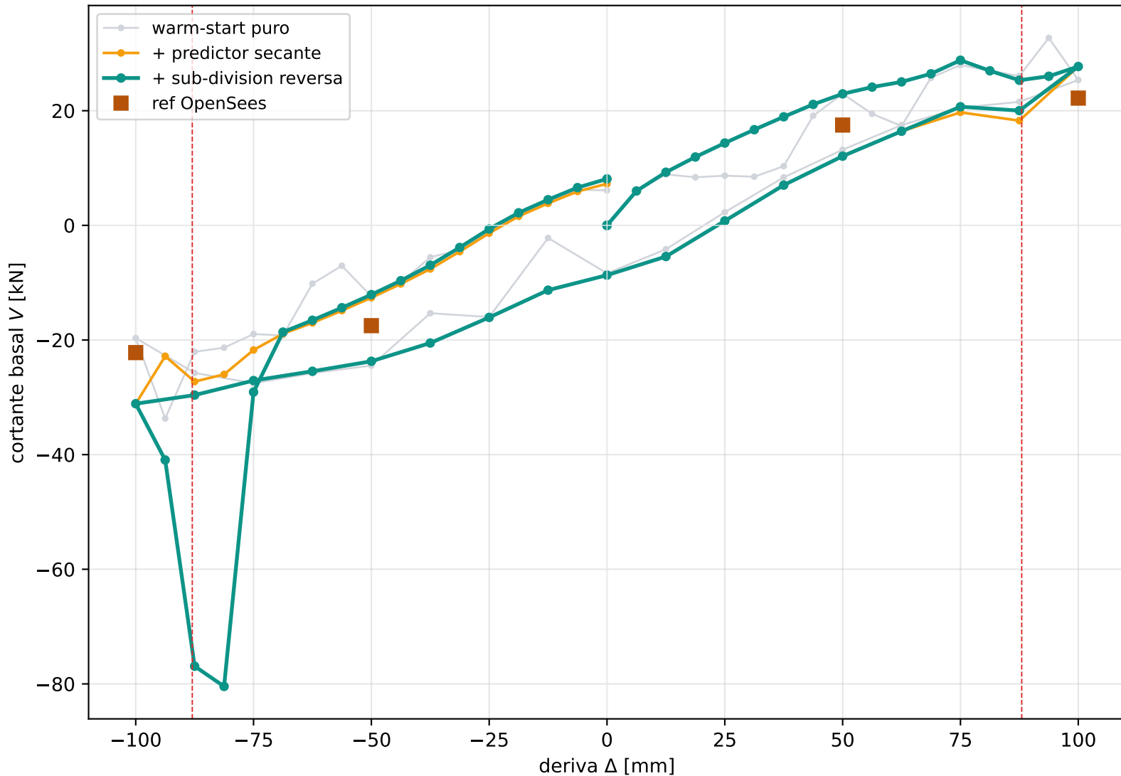
Ko-Bathe 3D AMPS=100 — limpieza del lazo por continuacion LM
