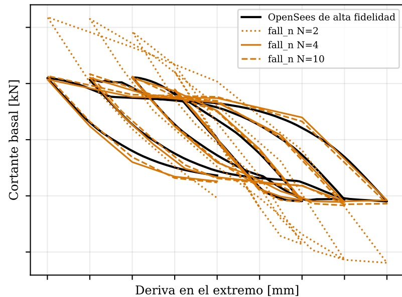
Gauss-Radau derecha
