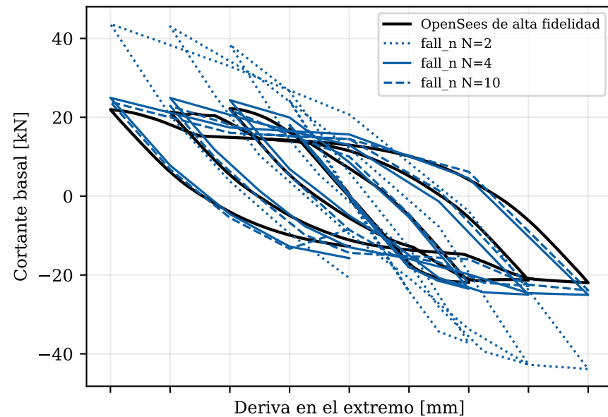
Gauss-Radau izquierda
