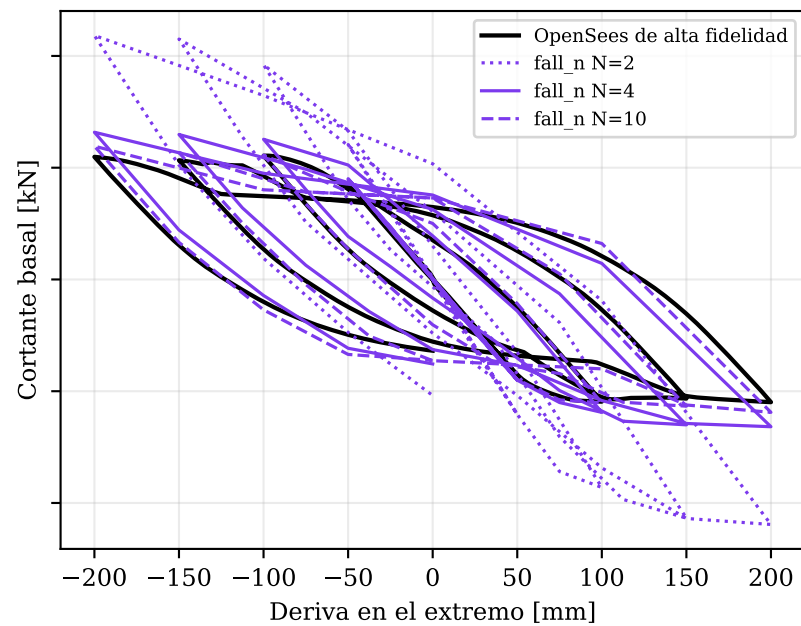
Gauss-Radau derecha
