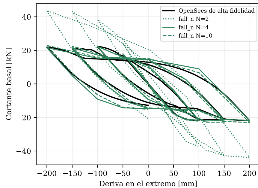
Gauss-Radau izquierda
