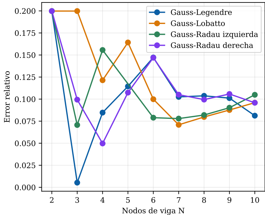
Coherencia física frente a OpenSees de alta fidelidad trabajo histerético total
