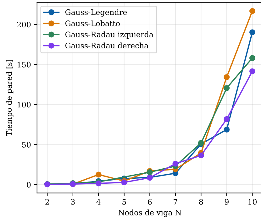
Tiempos de la matriz TimoshenkoBeamN
