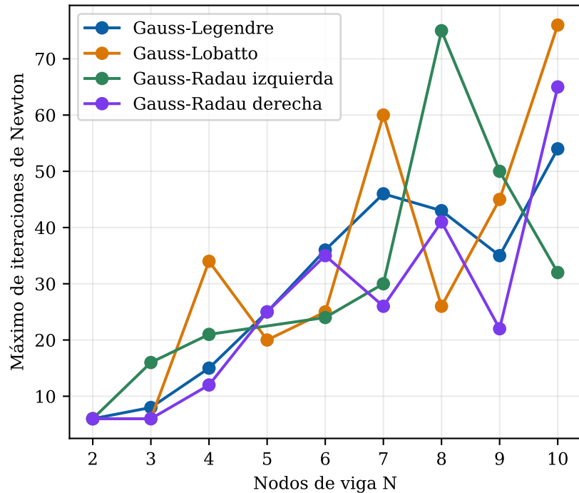
Convergencia de la matriz TimoshenkoBeamN
