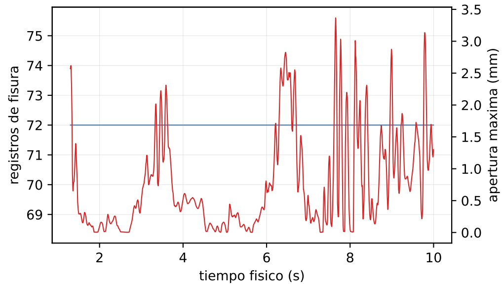
Evolucion local XFEM
