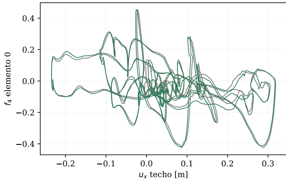
Lazo f_4-u_x
