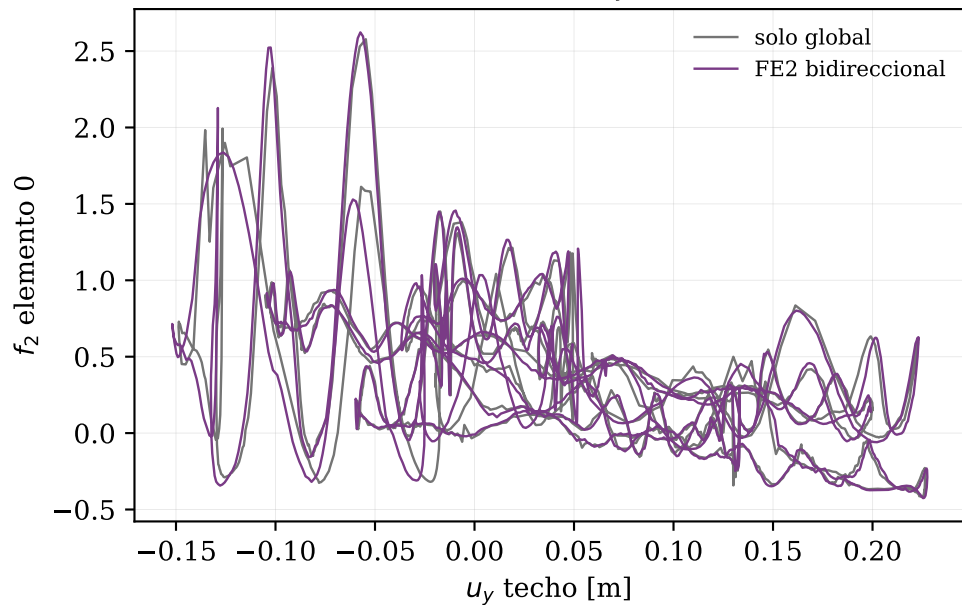
Lazo f_2-u_y
