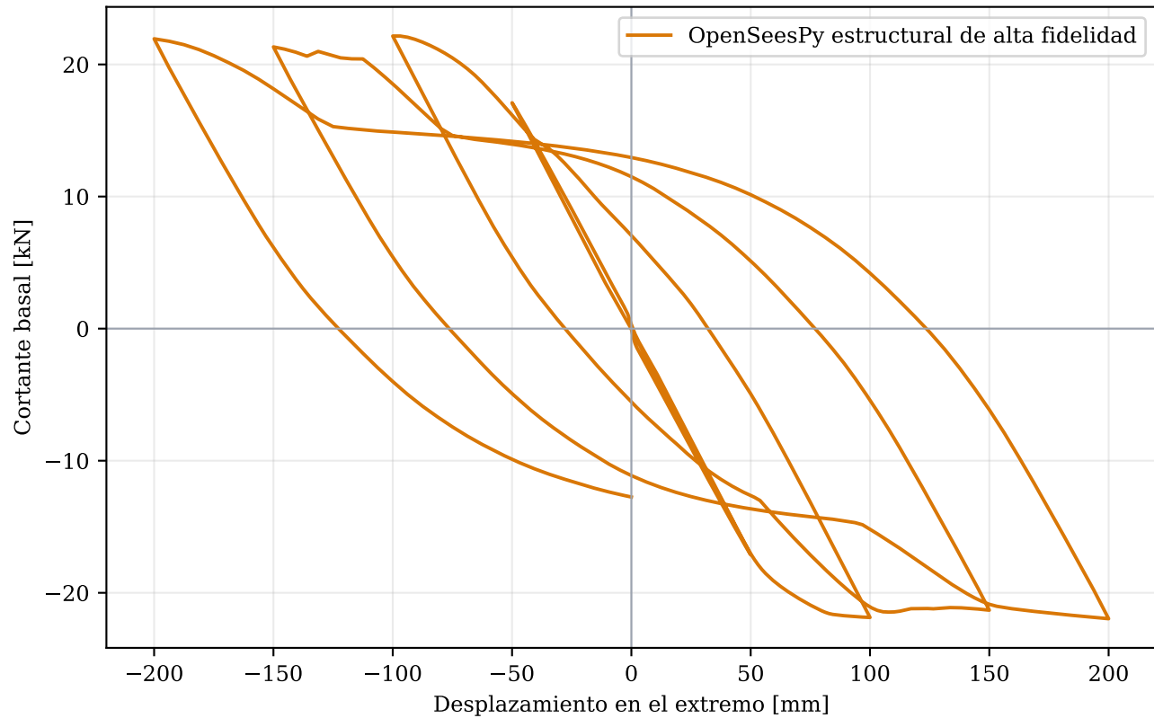
Referencia cíclica OpenSeesPy de alta fidelidad de la columna de concreto reforzado hasta 200 mm
