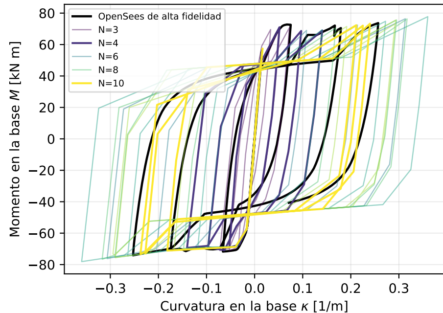
Gauss-Radau izquierda
