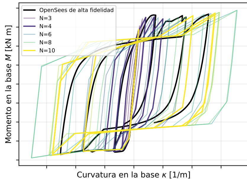
Gauss-Radau derecha
