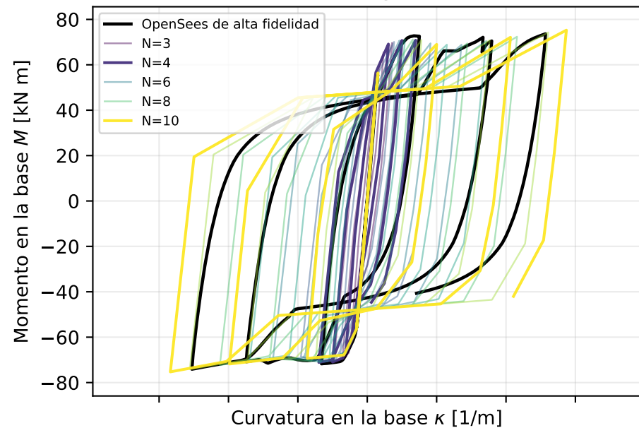
Gauss-Radau izquierda
