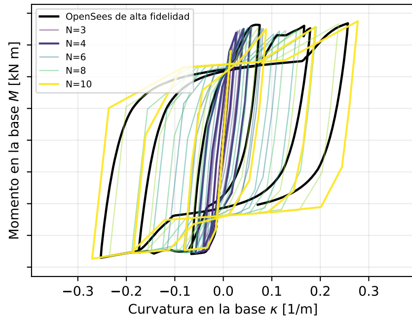
Gauss-Radau derecha
