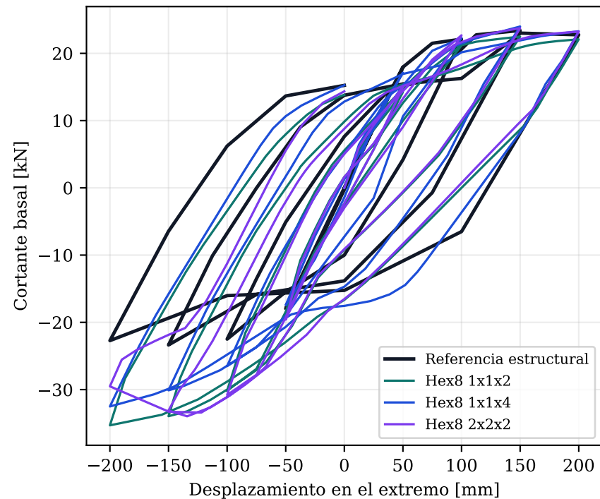
Histéresis cíclica, plano oblicuo con guarda
