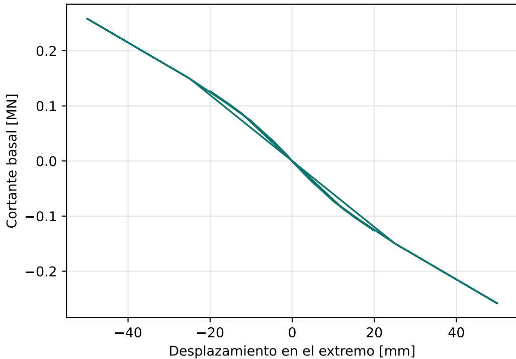
Sonda continua Ko-Bathe: 1x1x2 cíclica a 50 mm
