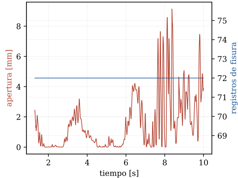
Respuesta local XFEM
