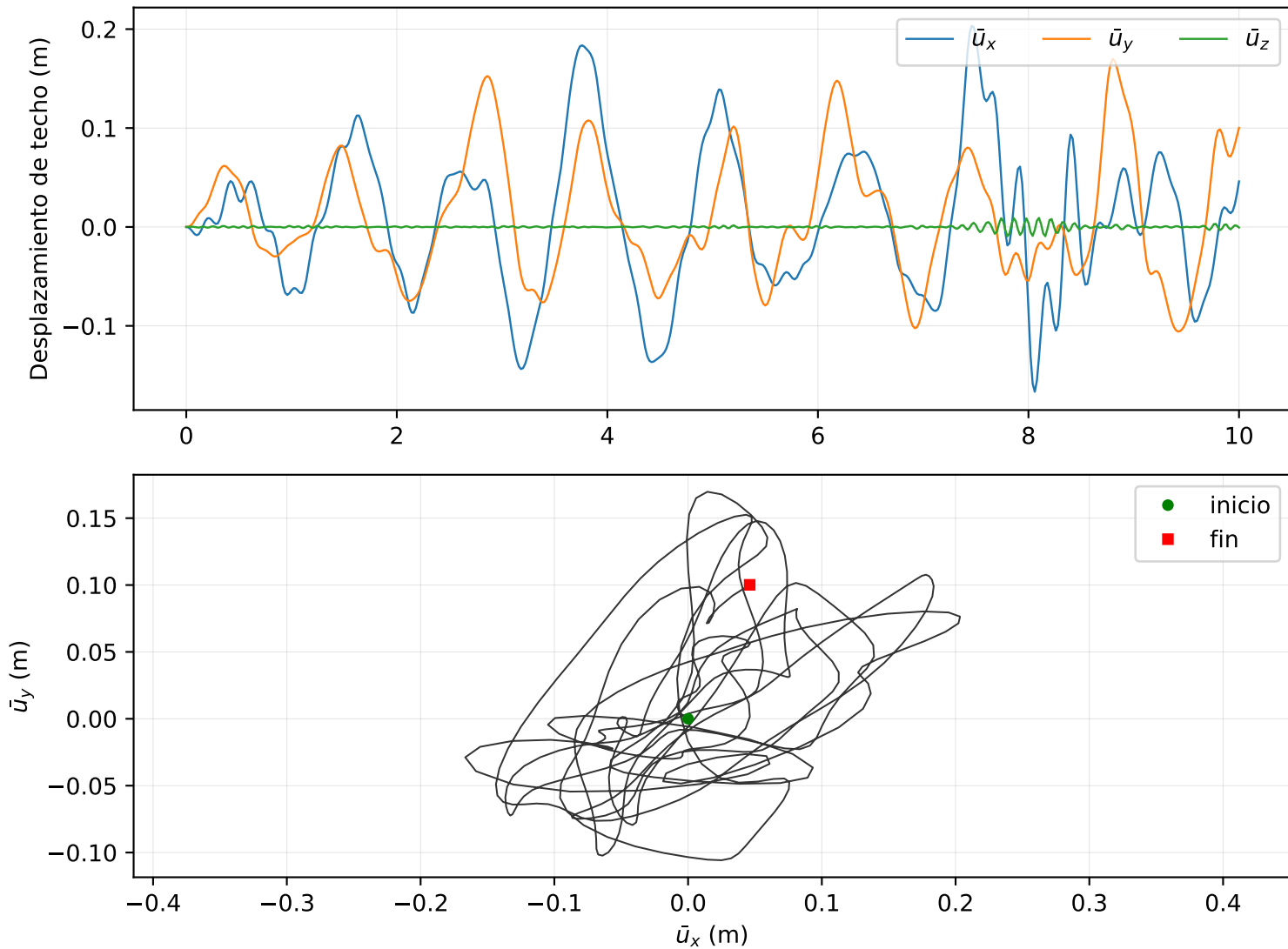
Edificio en L de 16 pisos, MYG004 físico escala=1: respuesta de control lineal
