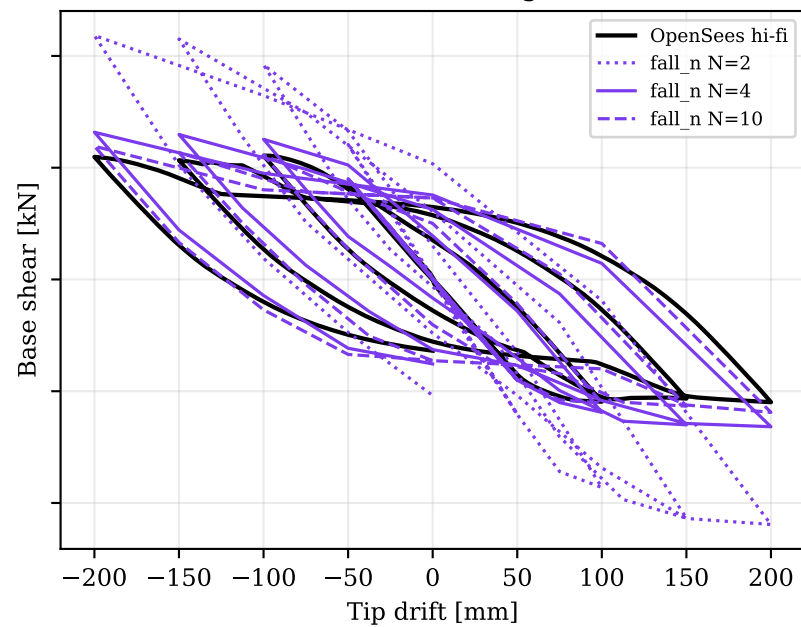
Gauss-Radau right
