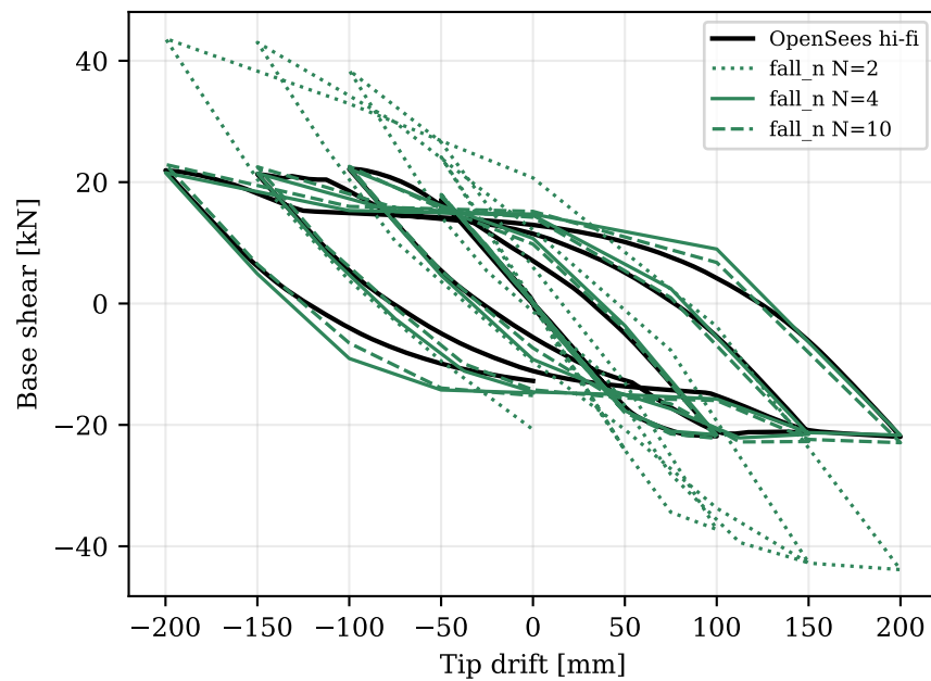
Gauss-Radau left
