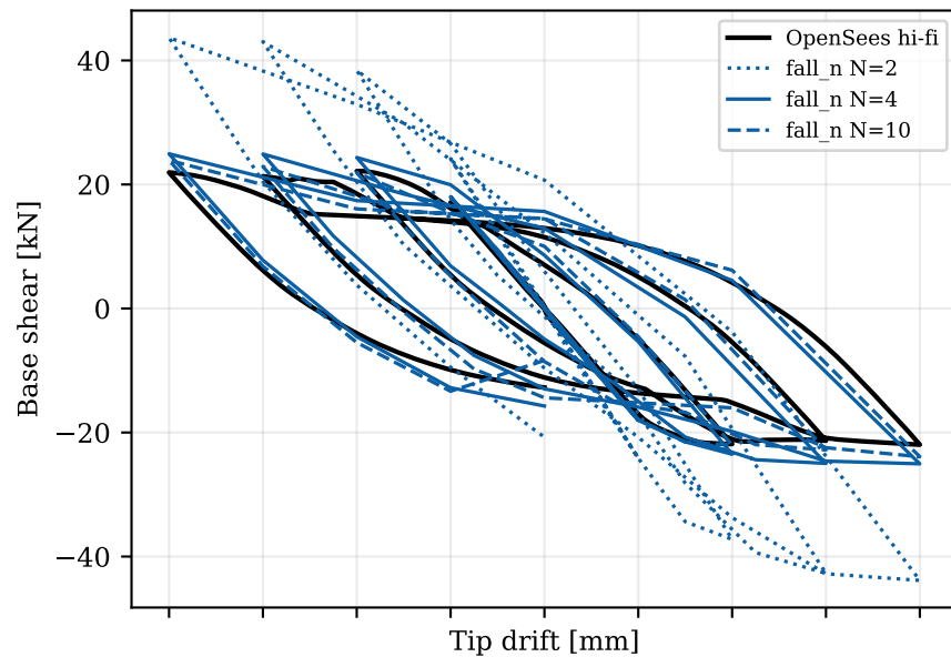
Gauss-Radau left
