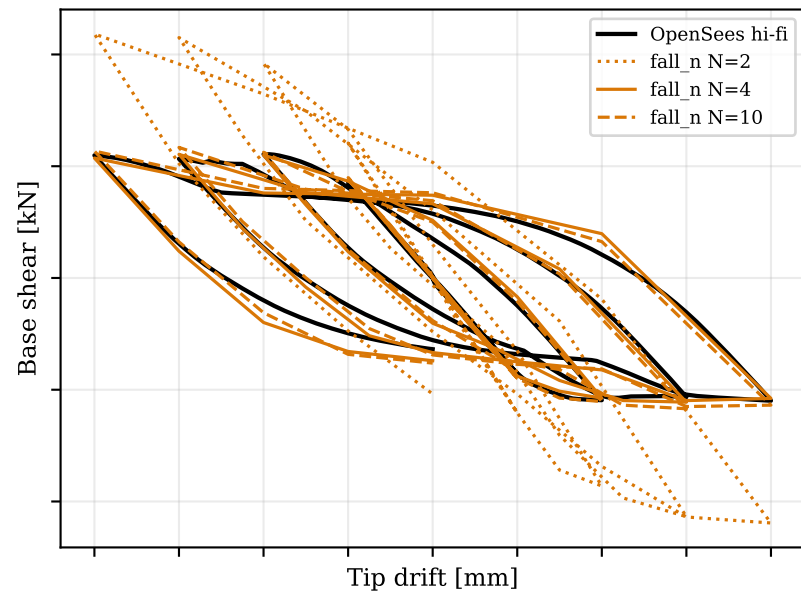
Gauss-Radau right
