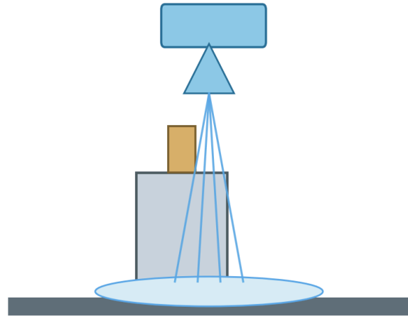
ALS
