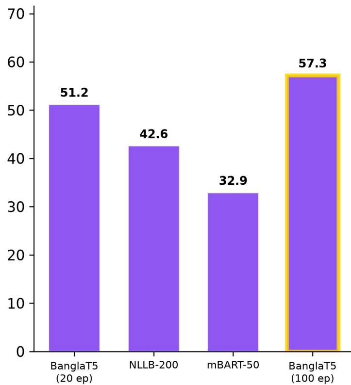
chrF++
