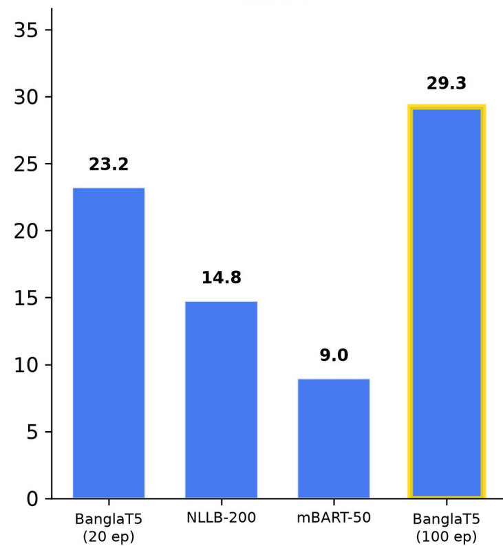
BLEU
