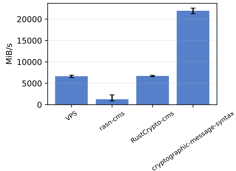
CMS RFC 4134 — parse
