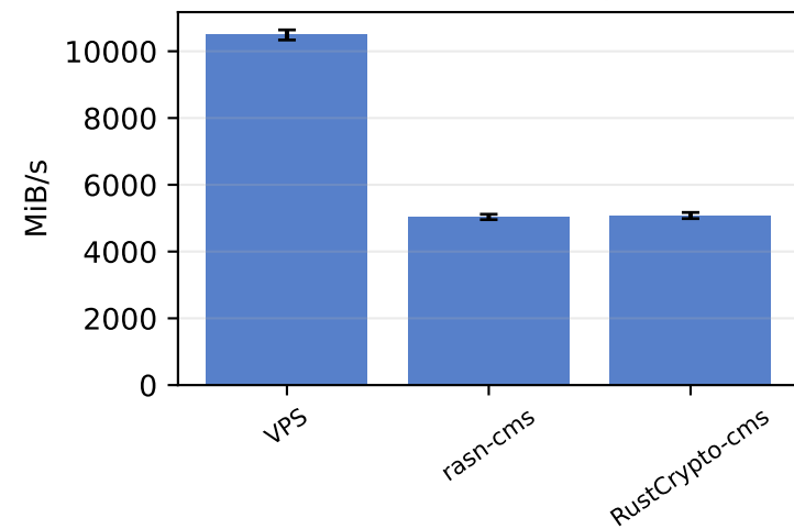
CMS EC DSS CADES — parse
