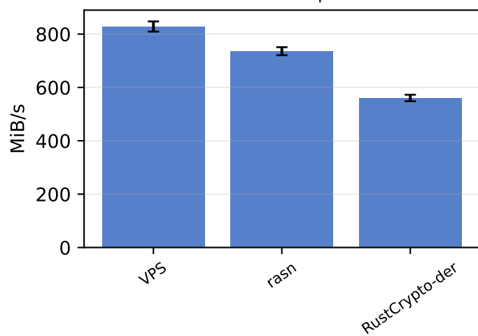
ASN.1 DER — parse
