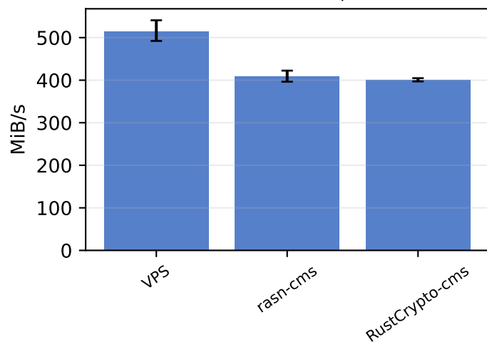
CMS RFC 4134 — parse
