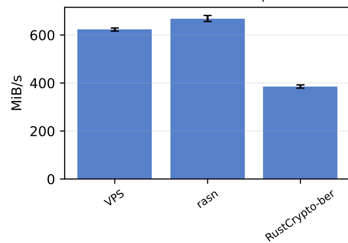
ASN.1 BER common — parse
