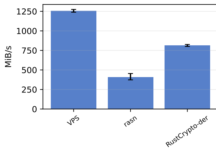
ASN.1 DER — serialize
