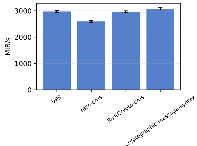
CMS EC DSS CADES — parse
