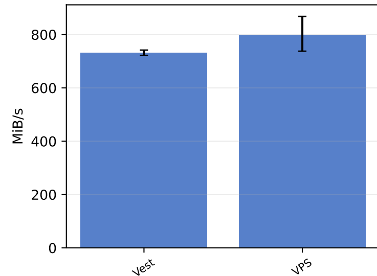
tls — parse
