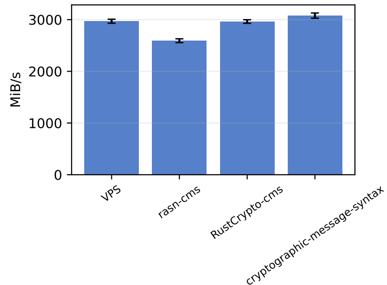
CMS EC DSS CADES — parse
