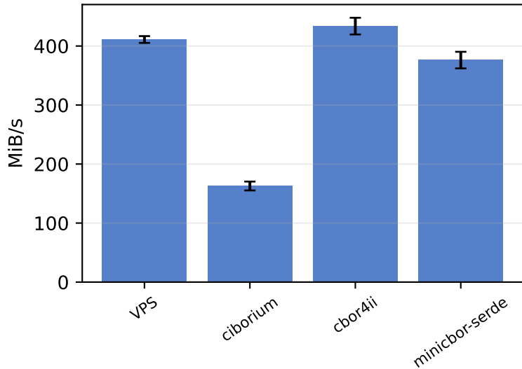
CBOR — parse
