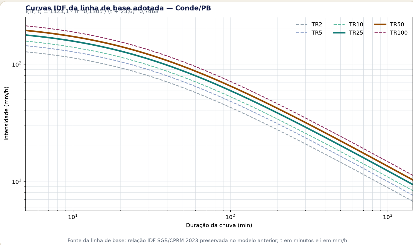
Figura 3.1 — Curvas IDF da linha de base adotada. TR25 e TR50 aparecem destacados por serem as recorrências usadas na primeira concepção; as demais curvas contextualizam a relação entre frequência e intensidade.
