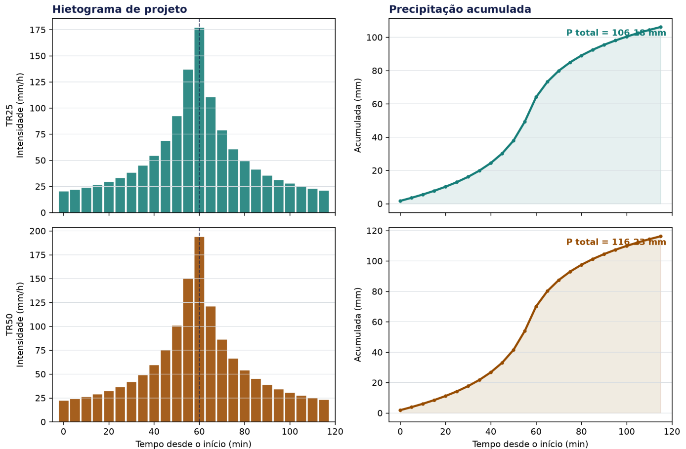
Figura 3.3 — Hietogramas de projeto tradicionais e precipitação acumulada. As barras representam as intensidades de cada intervalo de 5 minutos; as curvas mostram a soma acumulada utilizada como controle de consistência.
