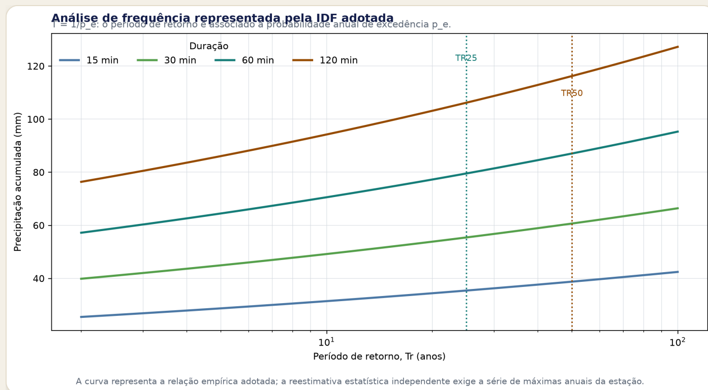
Figura 3.2 — Representação da análise de frequência embutida na equação IDF, com a precipitação acumulada variando com o período de retorno e a duração.
