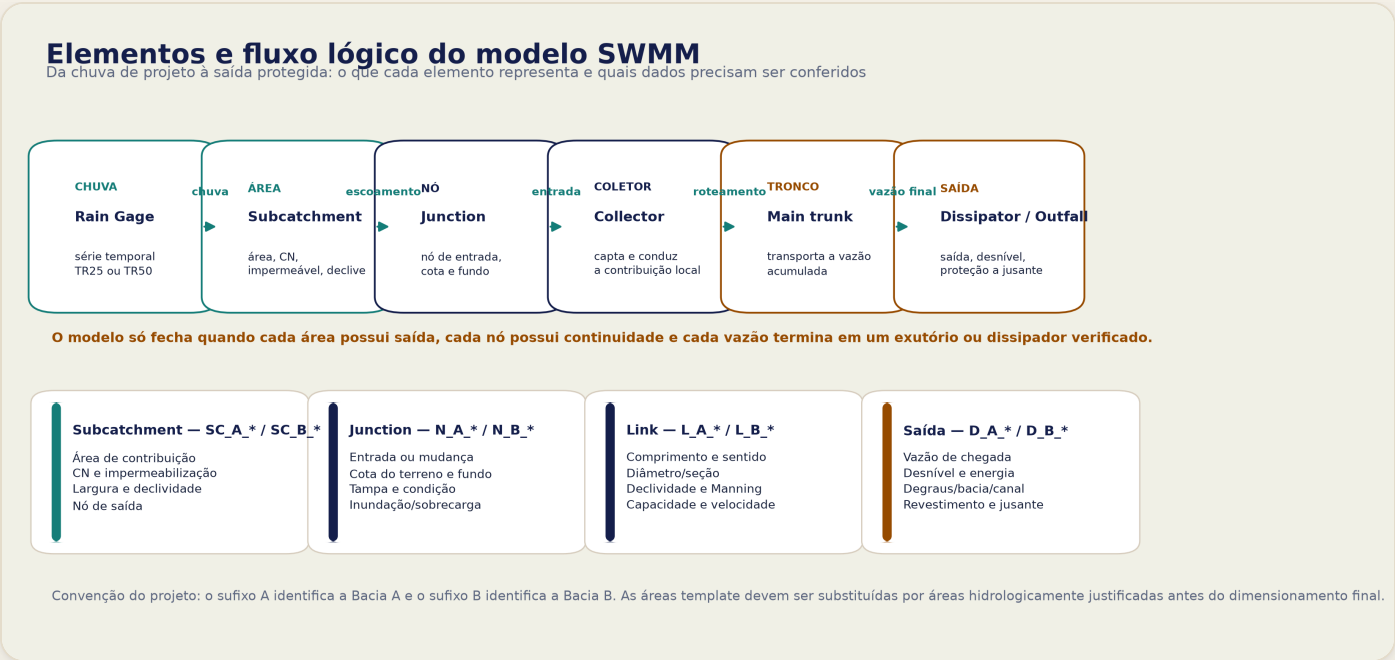
Figura 4.1 — Elementos e fluxo lógico do modelo SWMM. A chuva é aplicada às áreas de contribuição; o escoamento chega aos nós, percorre coletores e troncos e termina em dissipadores ou exutórios com condição de jusante verificada. Os identificadores distinguem as Bacias A e B.
