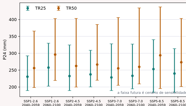
Figura 6.2 - Regra de chuva de projeto e tradução preliminar da incerteza climática para o dimensionamento. TR25 orienta coletores e bueiros; TR50 orienta troncos e dissipadores. O multiplicador de diâmetro é uma aproximação hidráulica para triagem.
