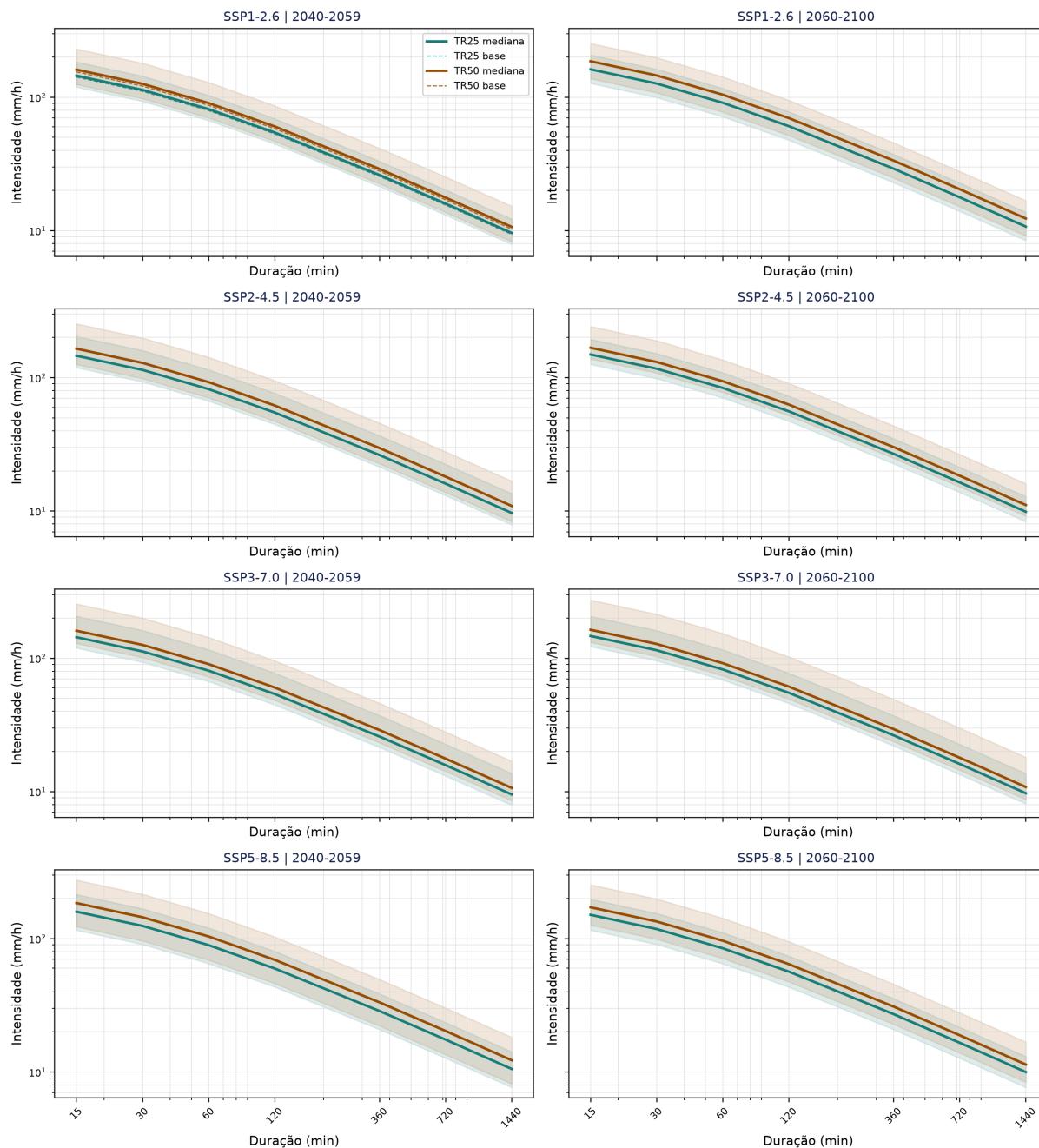
Figura 6.1 - Pannel de sensibilidade das IDFs para as Bacias A+B. As faixas P10-P90 expressam a dispersão do conjunto de modelos; as linhas tracejadas representam a IDF local de referência.
