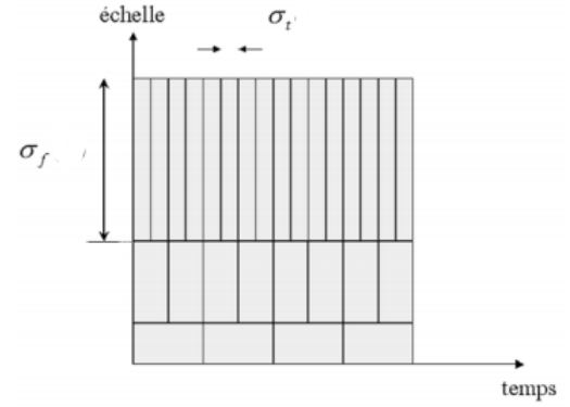
FIGURE 2.5 – Pavage temps-fréquence adapté aux transformées à ondelettes appelé pavage temps-échelle
