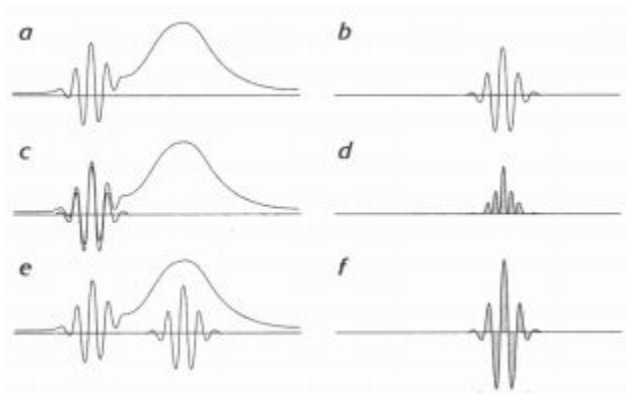
FIGURE 2.6 – Processus de Transformée à ondelettes
