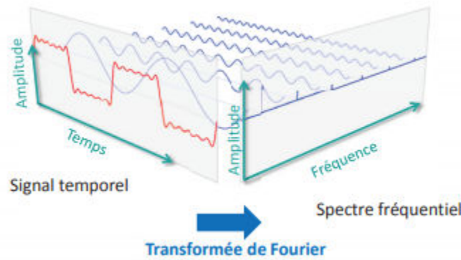
FIGURE 2.2 – Illustration de l'utilité de la transformée de Fourier, elle permet de passer du domaine temporel (à gauche) au domaine fréquentiel (à droite)
