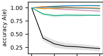
cifar100
