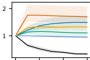
cub200
