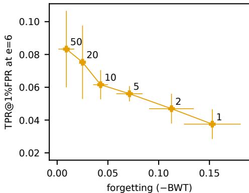
M5 exemplar replay (individual)
